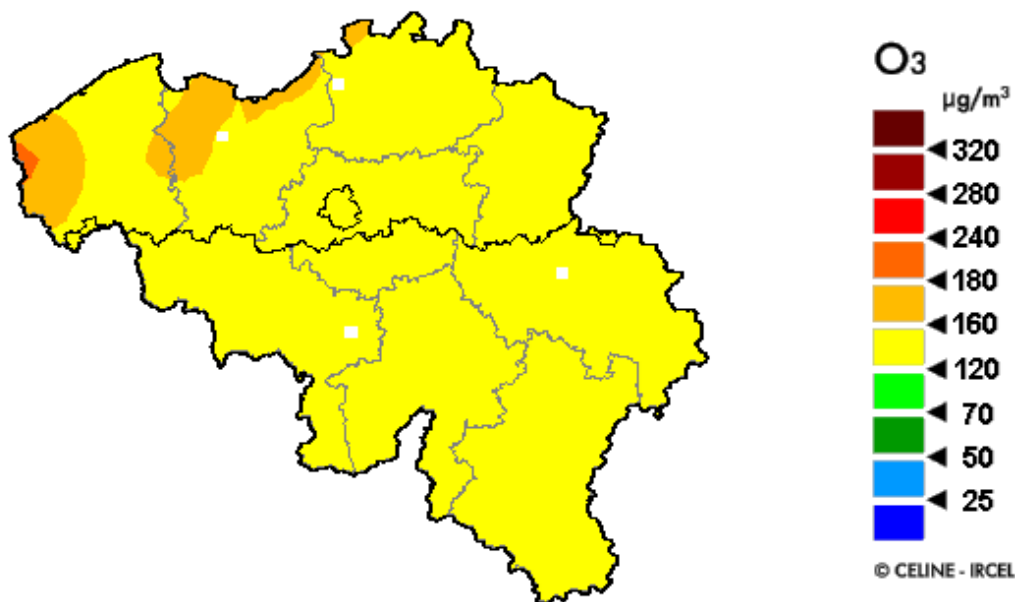
Verwachte hoogste uurgemiddelde ozonconcentraties overmorgen zondag 14 augustus 2022
