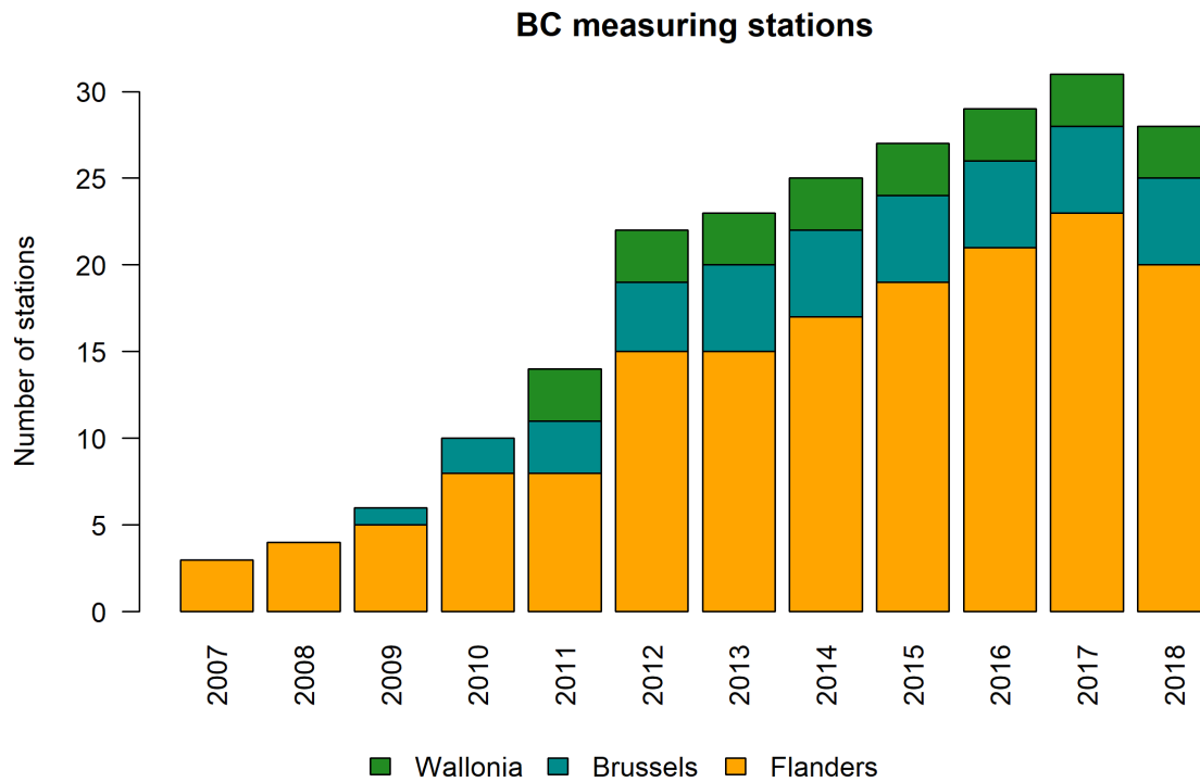
Figuur 27: Evolutie van het aantal BC meetstations in België.
