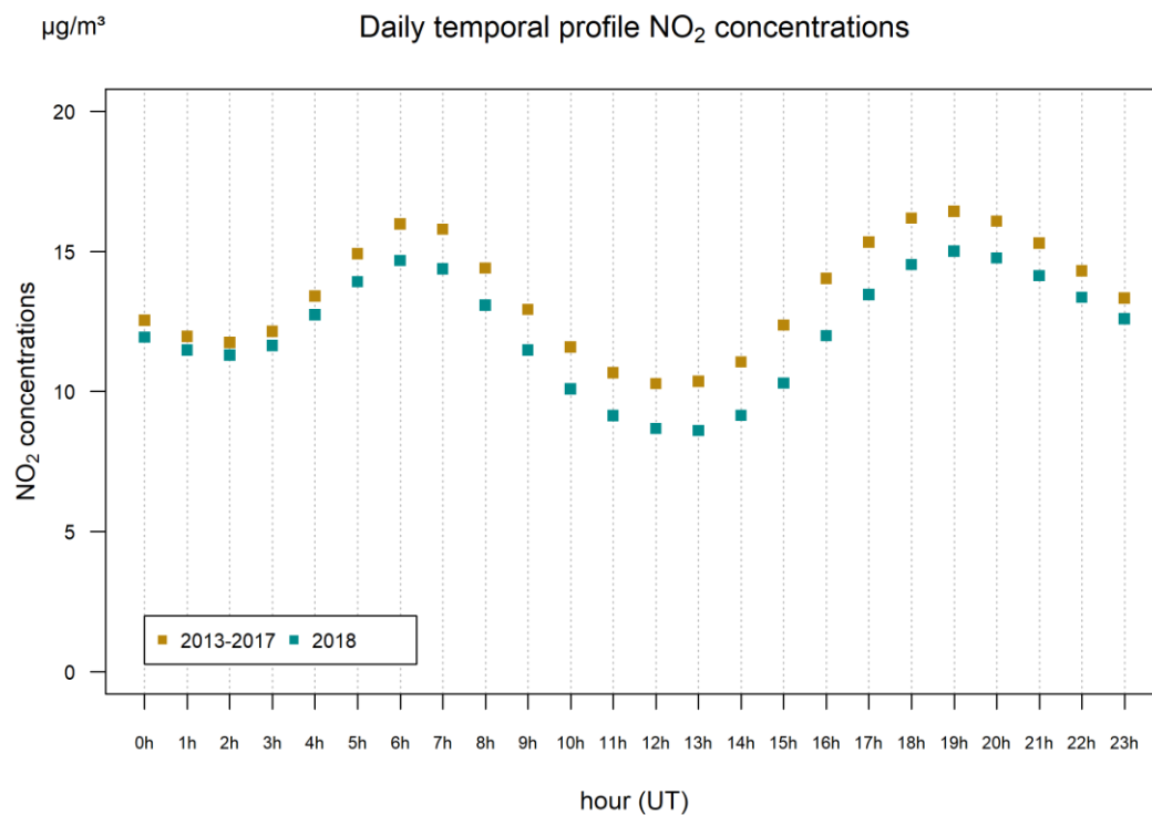
Figuur 35: Evolutie van de NO 2 -concentraties opgesplitst per uur.
