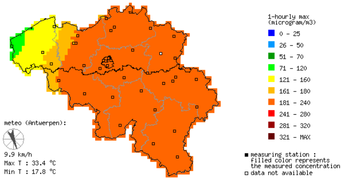
Figuur 8: Hoogste ozonconcentraties op 3 augustus 2018
