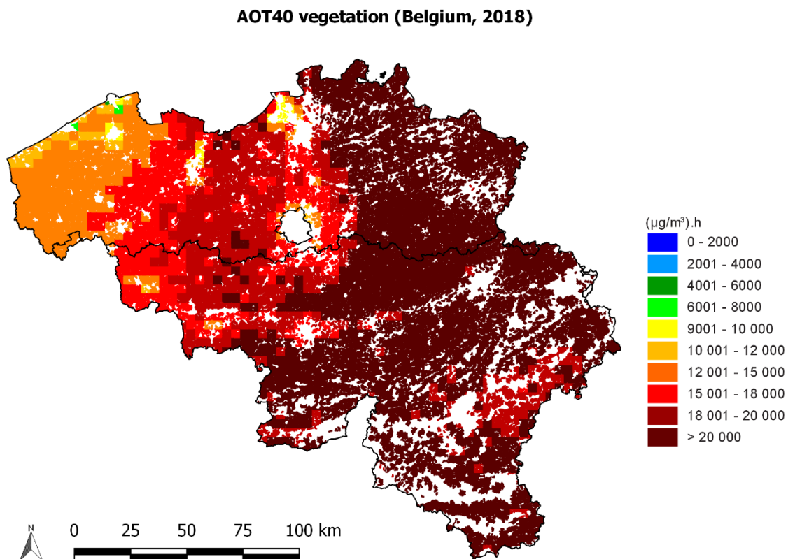
Figuur 47: Ruimtelijke spreiding van de overlast voor de vegetatie (AOT40 voor vegetatie) in 2018. ‘No data available’ betekent dat de data niet voldoen aan de criteria uit richtlijn 2008/50/EG annex VII voor het aggregeren van de meetgegevens. Alle data werden berekend op basis van de RIO-interpolatietechniek.
