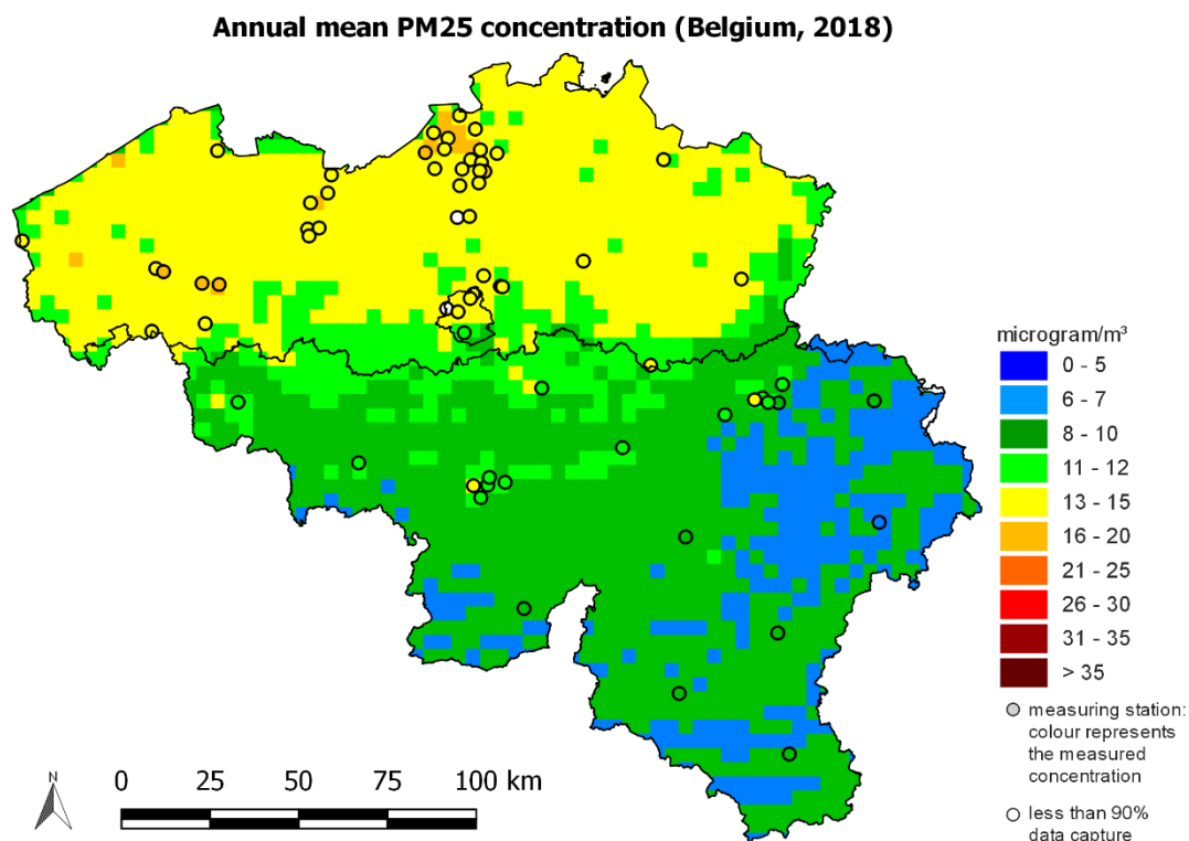
Figuur 21: Ruimtelijke spreiding van de jaargemiddelde PM 2,5 -concentratie in België in 2018. Alle data werden berekend op basis van de RIO-interpolatietechniek.
