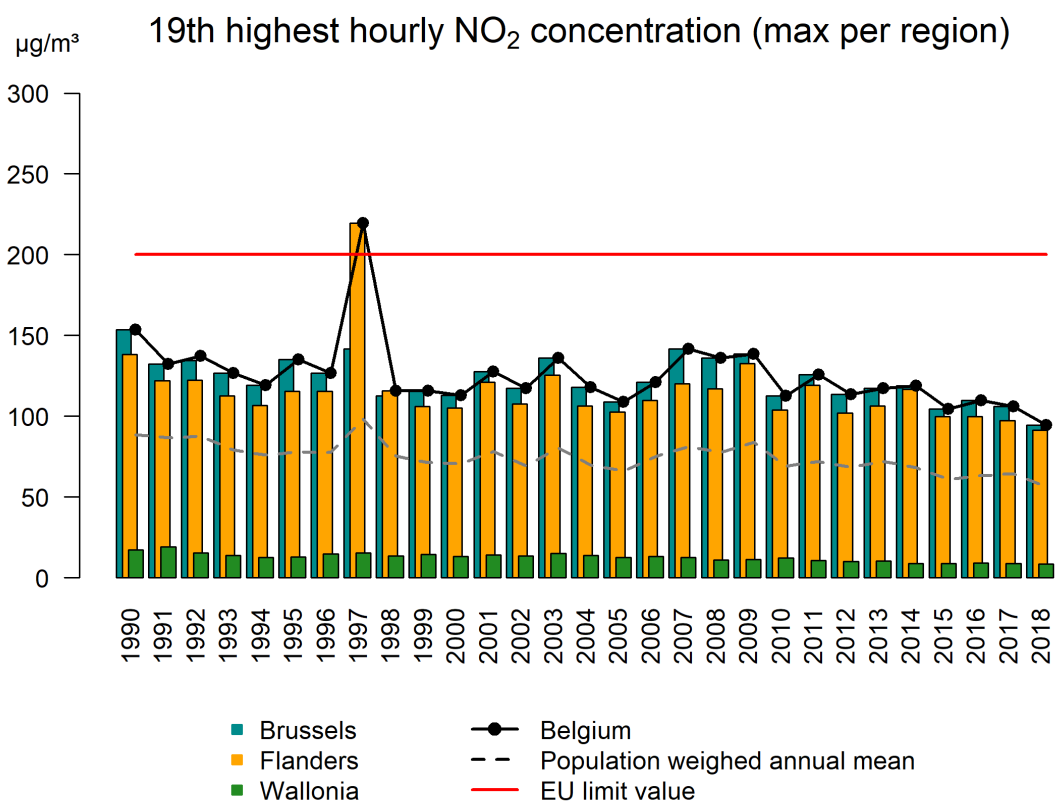
Figuur 39: Boxplot van de 19 de hoogste uurgemiddelde NO 2 -concentratie (µg/m 3 ) over de periode 1990-2018. Het ruimtelijke gemiddelde wordt door de blauwe cirkels weergegeven. Alle data werden berekend op basis van de RIO-interpolatietechniek.
