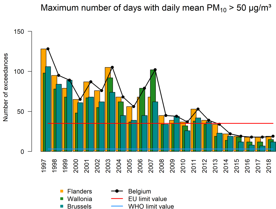
Figuur 17: Evolutie van het maximale aantal dagen per jaar waarop de daggemiddelde PM 10 -concentratie hoger was dan 50 µg/m 3 in België en de drie gewesten. Alle data werden berekend op basis van de RIO-interpolatietechniek.
