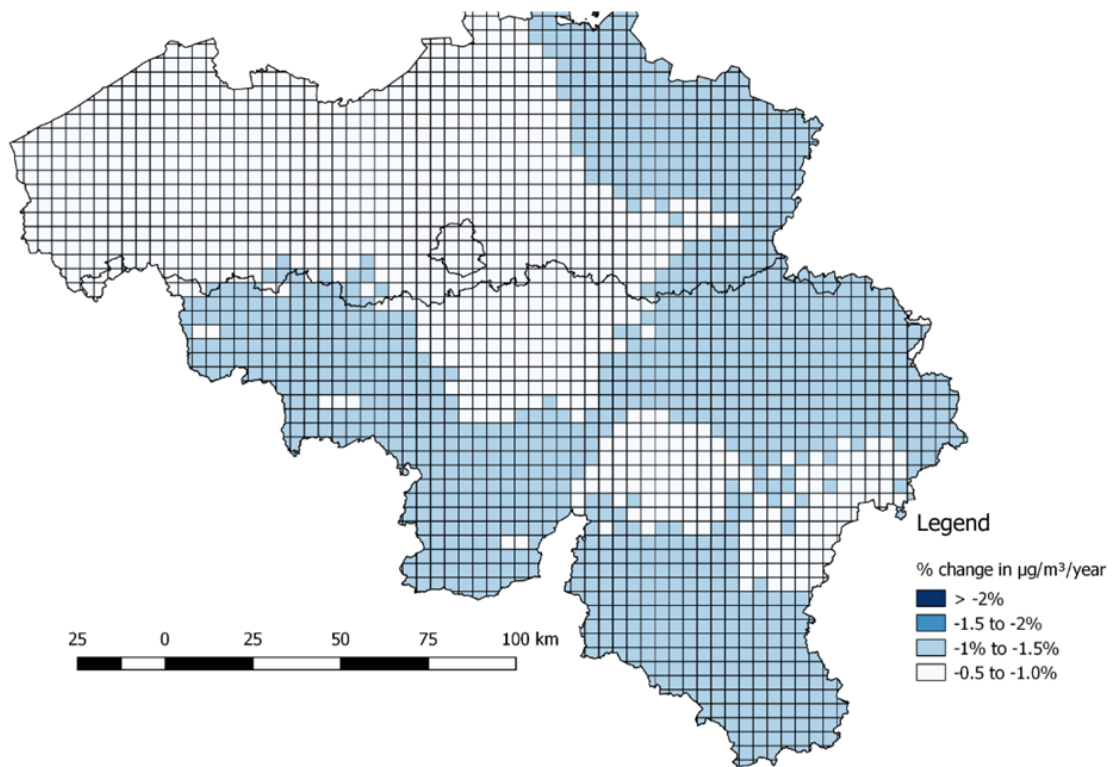
Figuur 36: Trend (%/jaar) van de jaargemiddelde NO 2 -concentraties in de periode 1990-2018. Alle data werden berekend op basis van de RIO-interpolatietechniek.
