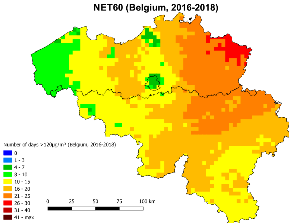
Figuur 43: Ruimtelijke spreiding van aantal dagen met hoogste 8-uurgemiddelde > 120 µg/m 3 , gemiddeld over 2016, 2017 en 2018. ‘No data available’ betekent dat de data niet voldoen aan de criteria uit richtlijn 2008/50/EG annex VII voor het aggregeren van de meetgegevens. Alle data werden berekend op basis van de RIO-interpolatietechniek.
