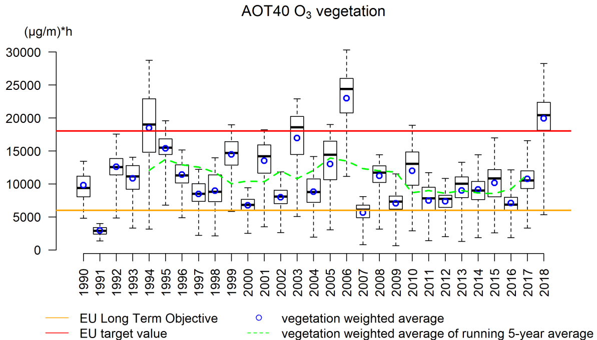
Figuur 49: Boxplots van de overlast voor de vegetatie (AOT40) in België (1991-2018). De vegetatiegewogen gemiddelden voor België worden weergegeven door de blauwe cirkels. De groene stippellijn geeft het vegetatiegewogen gemiddelde weer van de 5-jaargemiddelde AOT40. Alle data werden berekend op basis van de RIO-interpolatietechniek.
