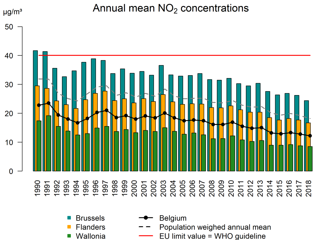
Figuur 33: Evolutie van het NO 2 -jaargemiddelde in België op basis van de RIO-interpolatietechniek.
