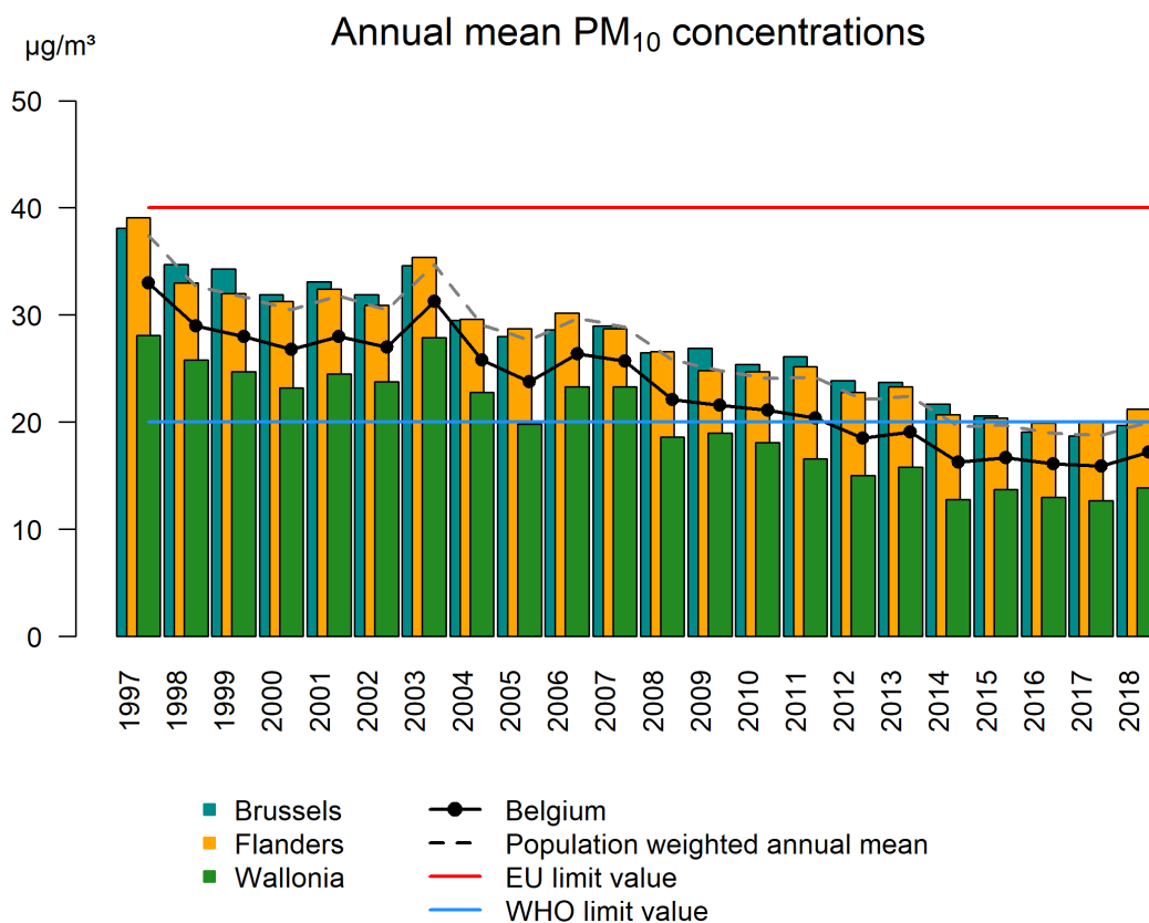
Figuur 12: Evolutie van de ruimtelijk gespreide jaargemiddelde PM 10 -concentratie in België en de drie gewesten, en het bevolkingsgewogen gemiddelde voor België. Alle data werden berekend op basis van de RIO-interpolatietechniek.
