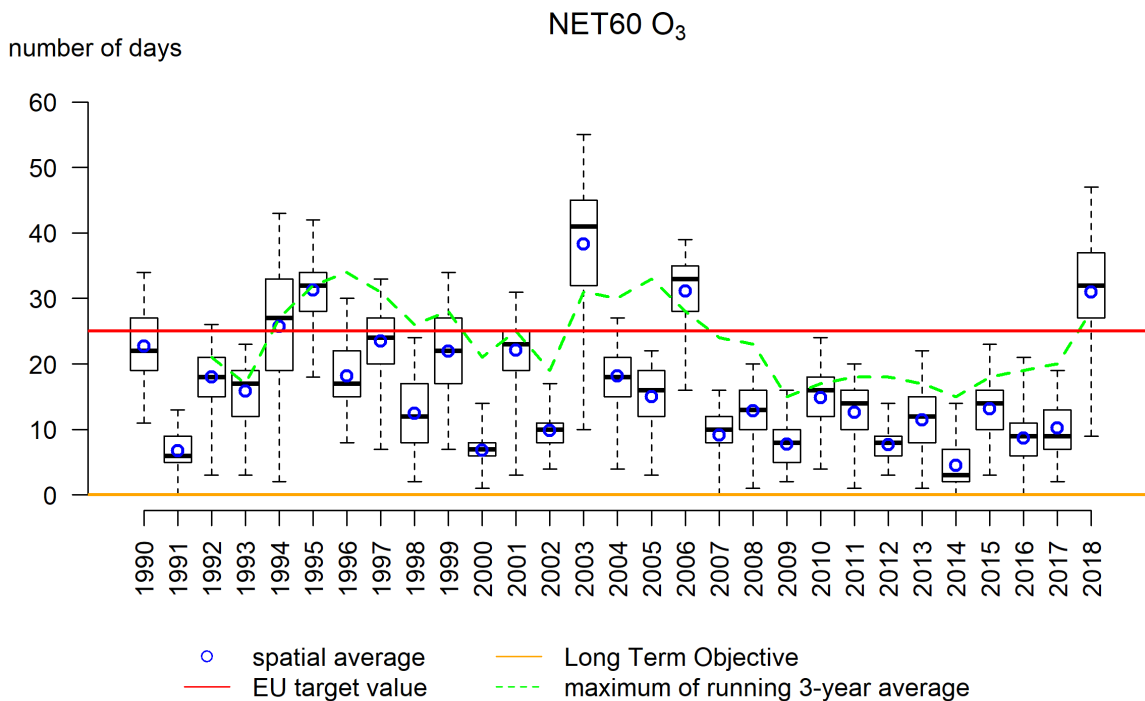
Figuur 44: Boxplots van aantal dagen met hoogste 8-uurgemiddelde ozonconcentraties > 120 µg/m 3 in België in de periode 1990-2018. Het ruimtelijke gemiddelde wordt weergegeven door de blauwe cirkels. De groene stippellijn geeft het maximum van het 3-jaargemiddelde aantal overschrijdingsdagen in België weer. Alle data werden berekend op basis van de RIO-interpolatietechniek.
