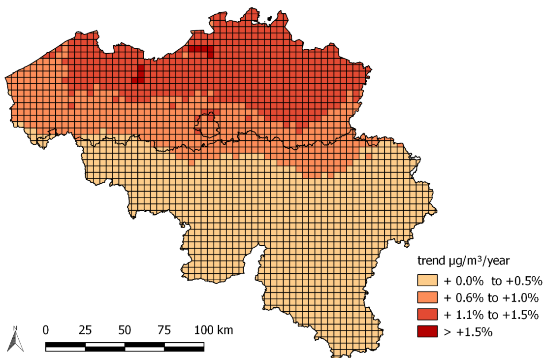
Figuur 56: Ruimtelijke trend in jaargemiddelde O 3 -concentratie (µg/m 3 /jaar) over de periode 1990-2018. De data voor de trendanalyse werden gegenereerd op basis van de RIO-interpolatietechniek.
