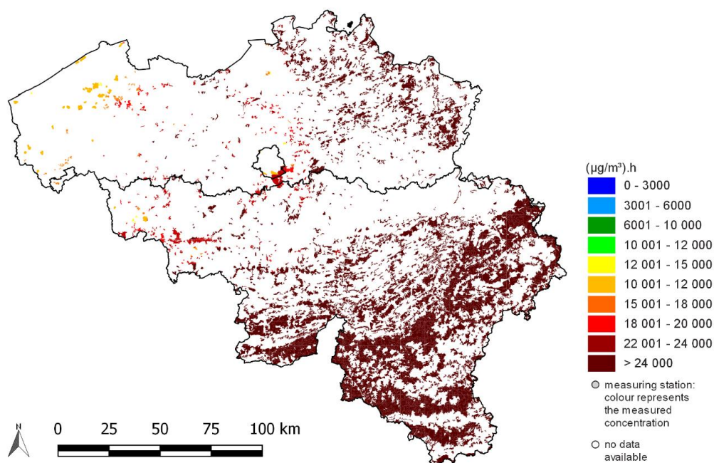
Figuur 50: Ruimtelijke spreiding van de ozonoverlast voor bossen (AOT40 voor bossen), 2018. ‘No data available’ betekent dat de data niet voldoen aan de criteria uit richtlijn 2008/50/EG annex VII voor het aggregeren van de meetgegevens. Alle data werden berekend op basis van de RIO-interpolatietechniek.
