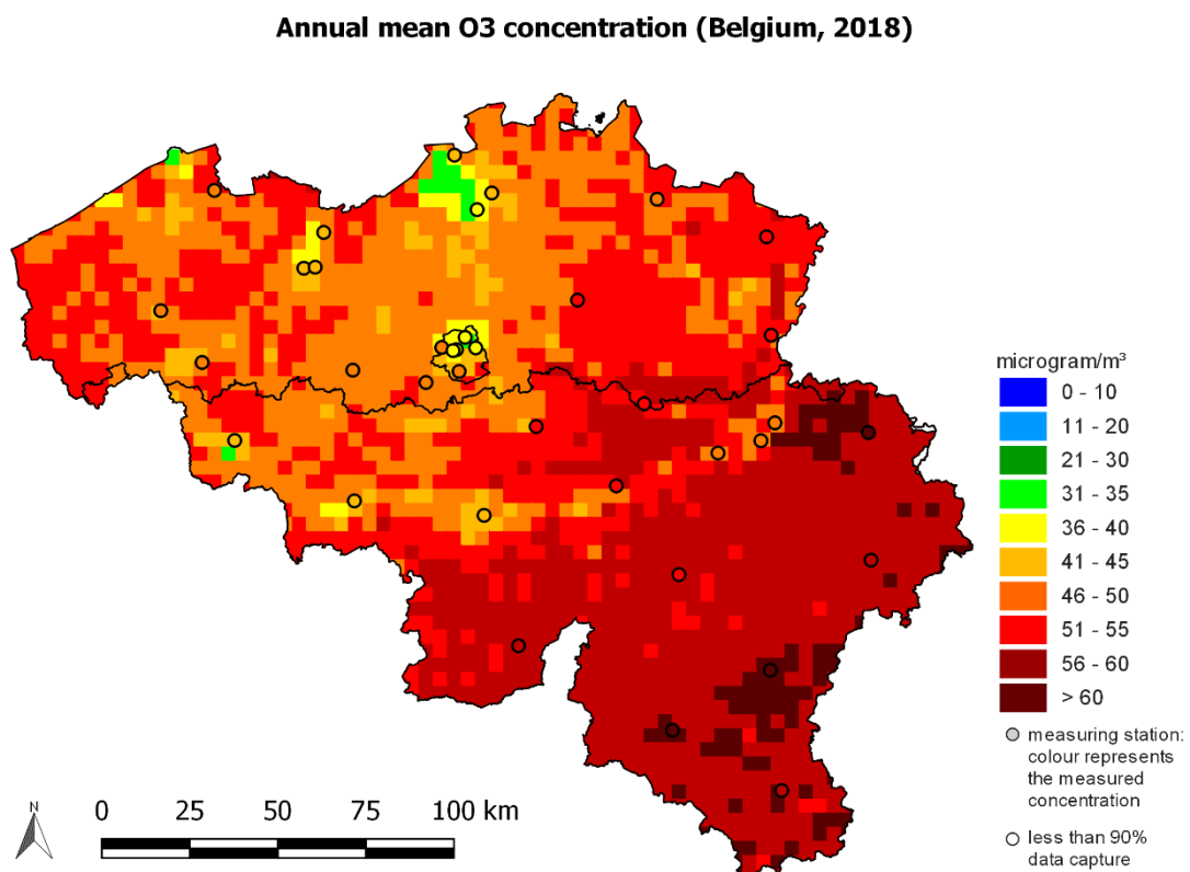
Figuur 52: Ruimtelijke spreiding van de O 3 -jaargemiddelde concentraties in België, 2018. Alle data werden berekend op basis van de RIO-interpolatietechniek.
