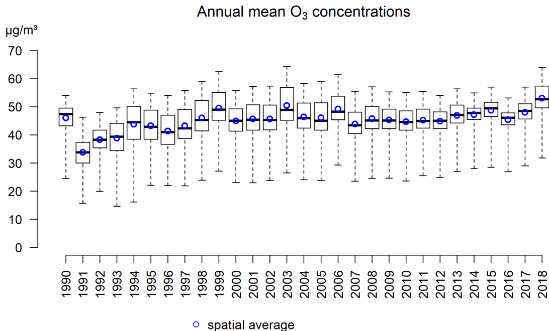
Figuur 54: Boxplot van jaargemiddelde O 3 -concentraties over de periode 1990-2018. Het ruimtelijk gemiddelde wordt weergegeven door de blauwe cirkels. Alle data werden berekend op basis van de RIO-interpolatietechniek.
