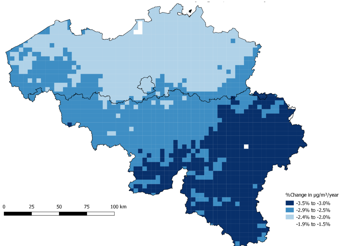
Figuur 13: Ruimtelijke trend in jaargemiddelde PM 10 -concentraties (%jaar). Alle data werden berekend op basis van de RIO-interpolatietechniek.
