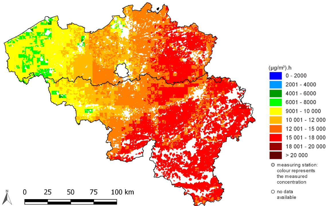
Figuur 48: Ruimtelijke spreiding van de overlast voor de vegetatie (AOT40 voor vegetatie), 5-jaargemiddelde 2014-2018. 'No data available' betekent dat de data niet voldoen aan de criteria uit richtlijn 2008/50/EG annex VII voor het aggregeren van de meetgegevens. Alle data werden berekend op basis van de RIO-interpolatietechniek.
