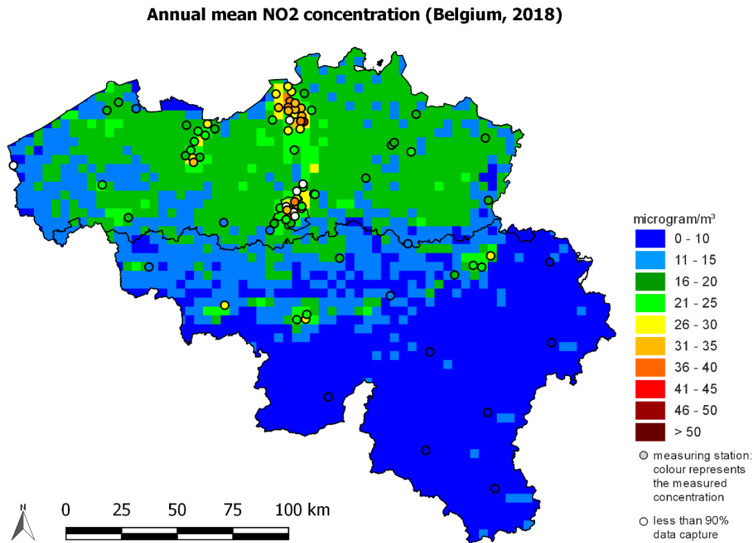
Figuur 30: Ruimtelijke spreiding van het \text{NO}_2 -jaargemiddelde in 2017. Alle data werden berekend op basis van de RIO-interpolatietechniek.
