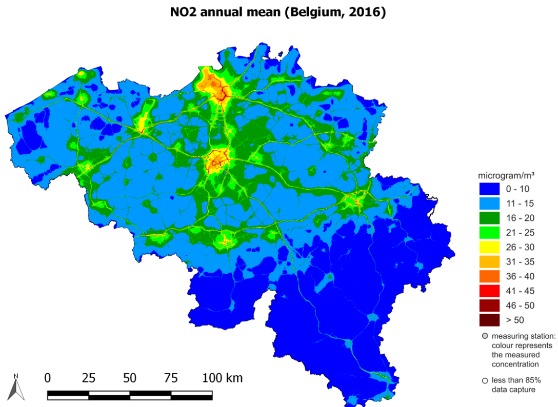
Figuur 60: RIO-IFDM-kaart van België voor de daggemiddelde NO 2 -concentraties op 28 maart 2014
