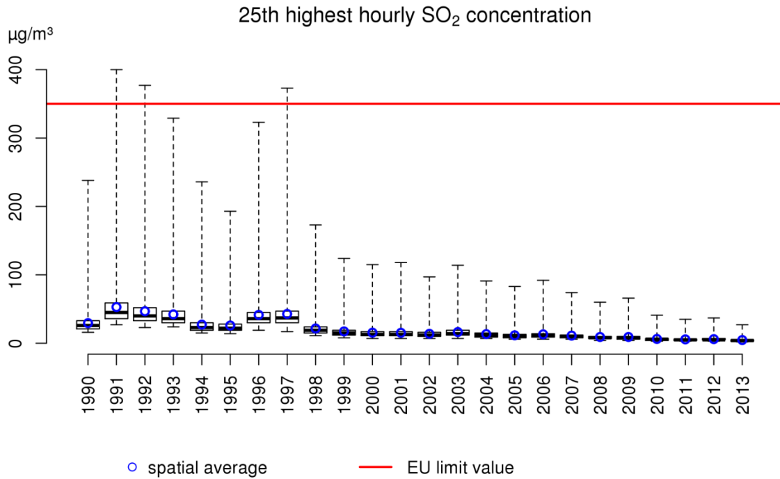
Figuur 58: Boxplot van de 25e hoogste uurgemiddelde SO 2 -concentratie over de periode 1990-2013 in België op basis van de RIO-interpolatietechniek.
