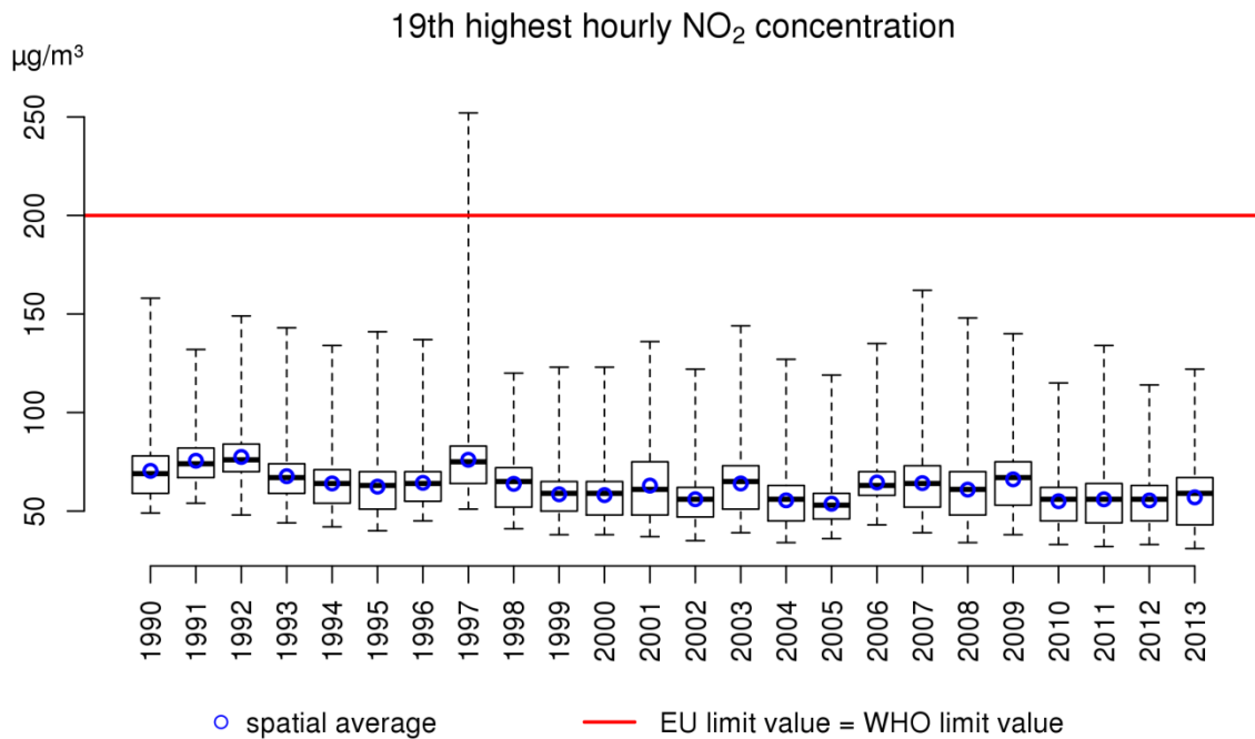
Figuur 35: Boxplot van de 19 de hoogste uurgemiddelde NO 2 -concentratie (µg/m 3 ) over de periode 1990-2013. Het ruimtelijke gemiddelde wordt door de blauwe cirkels weergegeven. Alle data werden berekend op basis van de RIO-interpolatietechniek.
