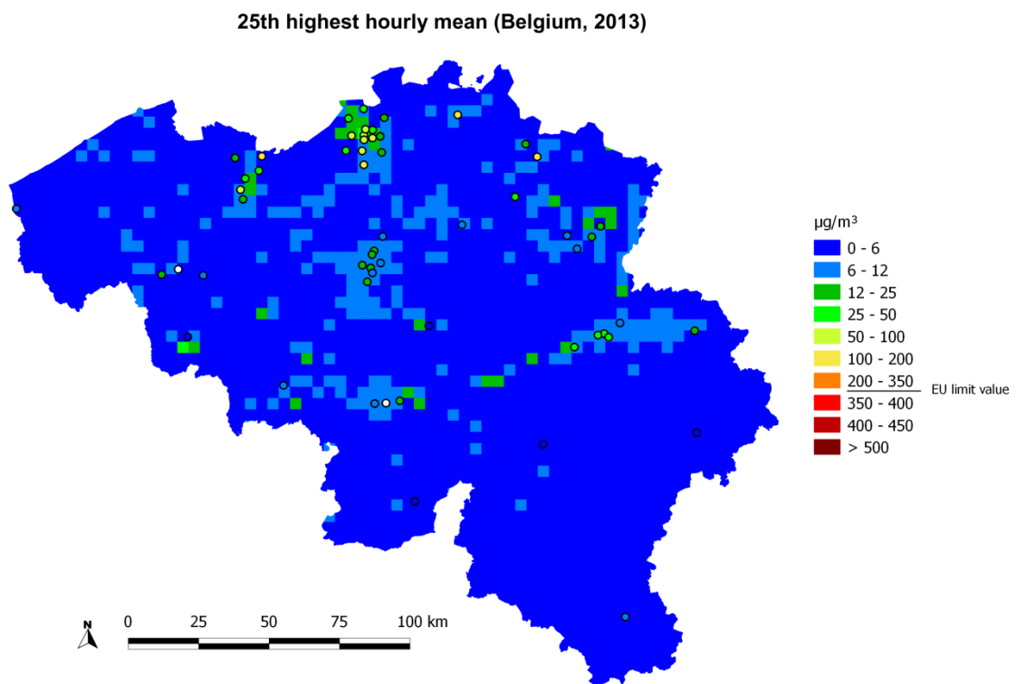
Figuur 56: 25e hoogste uurgemiddelde SO 2 -concentratie in 2013. Alle data werden berekend op basis van de RIO-interpolatietechniek.
