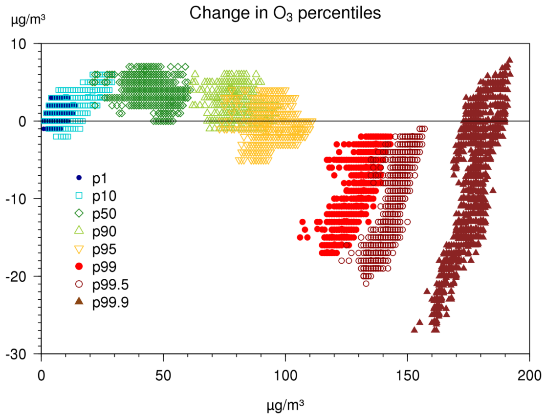
Figuur 54. Verandering in O 3 -percentielen tussen de periode 1990-2001 en 2002-2013 in functie van de percentielwaarden in de periode 2002-2013 voor alle RIO-gridcellen. De data (uurgemiddelde ozonconcentraties) werden gegenereerd op basis van de RIO-interpolatietechniek. De verschillende kleuren geven de verschillende percentielwaarden aan
