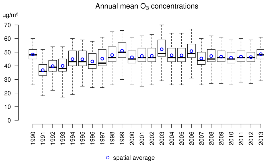
Figuur 51: Boxplot van jaargemiddelde O 3 -concentraties over de periode 1990-2013. Het ruimtelijk gemiddelde wordt weergegeven door de blauwe cirkels. Alle data werden berekend op basis van de RIO-interpolatietechniek.
