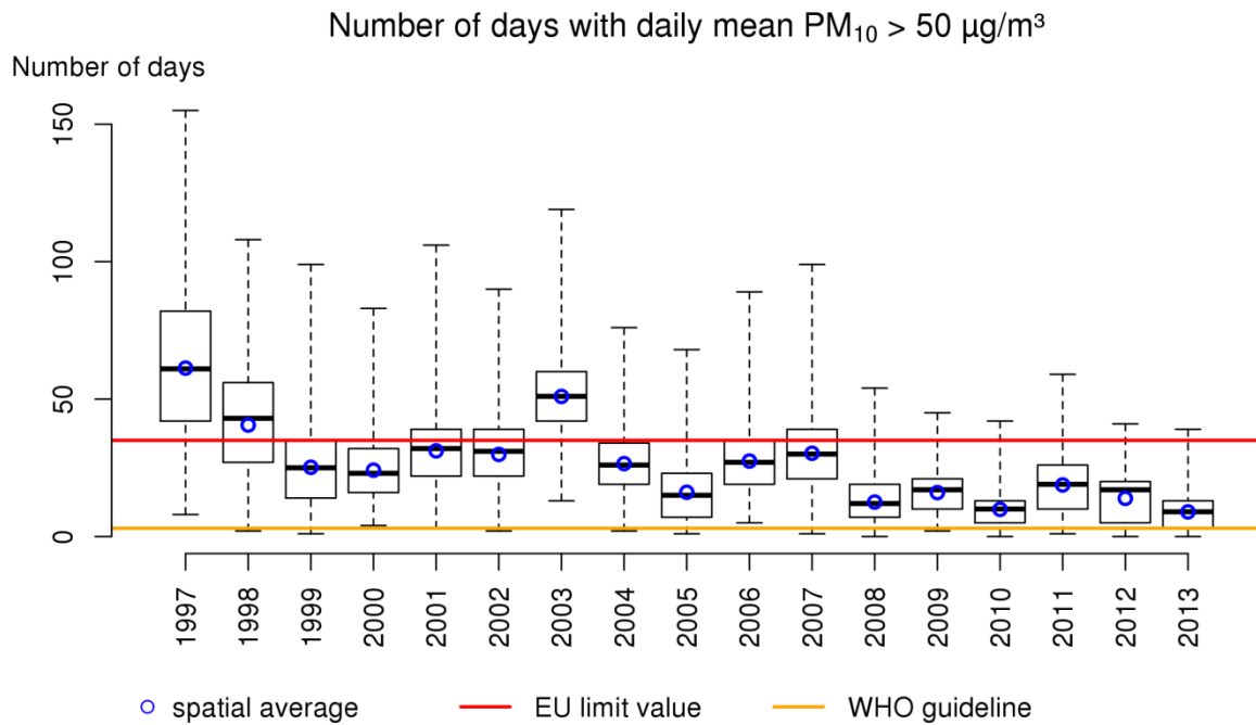
Figuur 14: Boxplot van het aantal dagen per jaar waarop de daggemiddelde PM_{10} -concentraties hoger was dan 50 \mu g/m^3 . Het ruimtelijk gemiddelde wordt weergegeven door de blauwe cirkels. Alle data werden berekend op basis van de RIO-interpolatietechniek.
