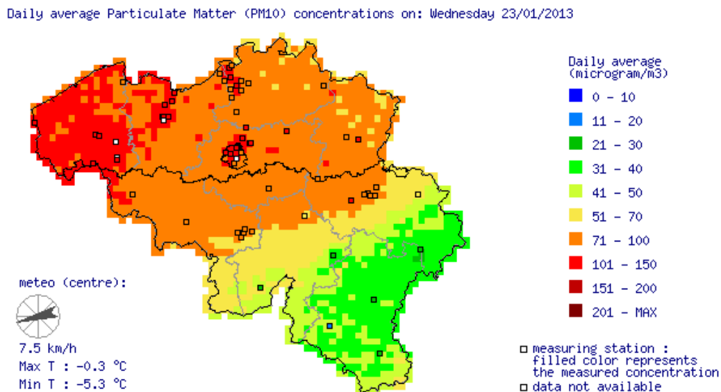
Figuur 5: Daggemiddelde fijnstofconcentratie op 23 januari 2013.
