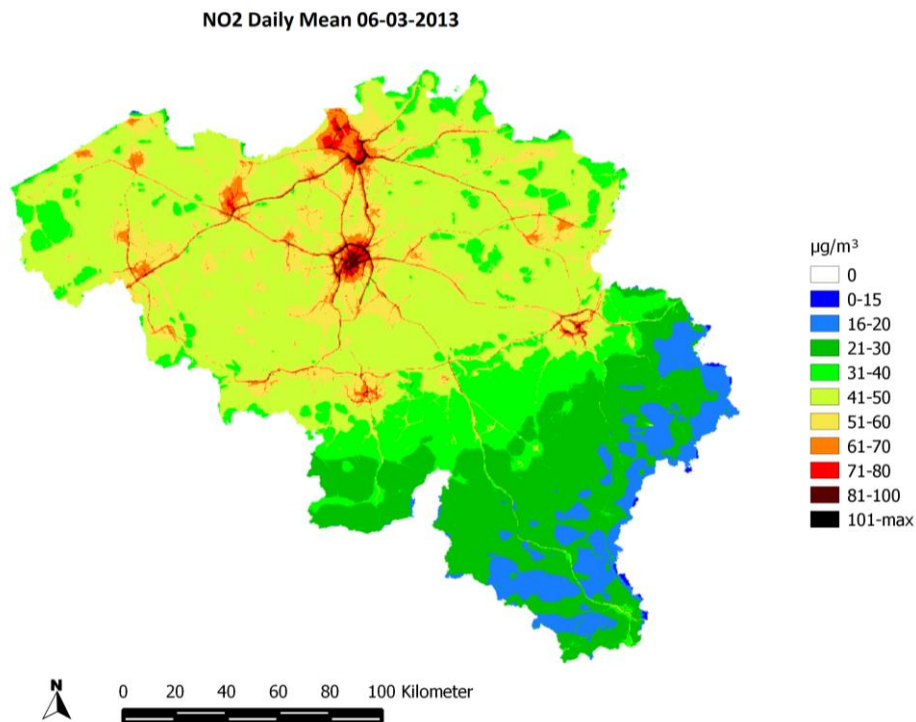
Figuur 61: RIO-IFDM-kaart van België voor de daggemiddelde NO 2 -concentraties op 6 maart 2013
