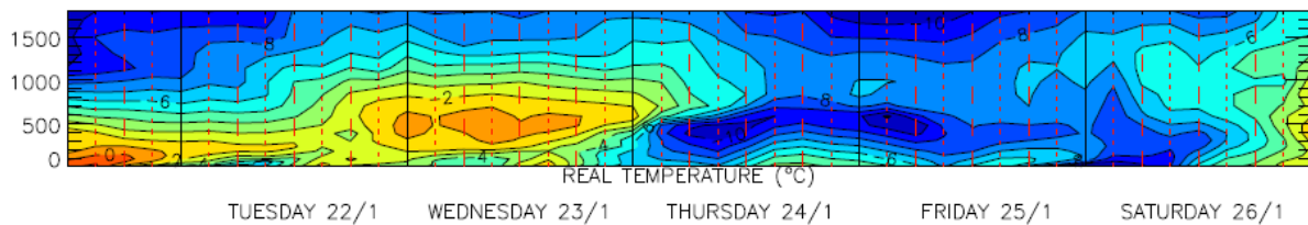
Figuur 4: ECMWF voorspelling voor de temperatuur in functie van de hoogte ( y). Op 23 januari is een temperatuursinversie duidelijk zichtbaar.
