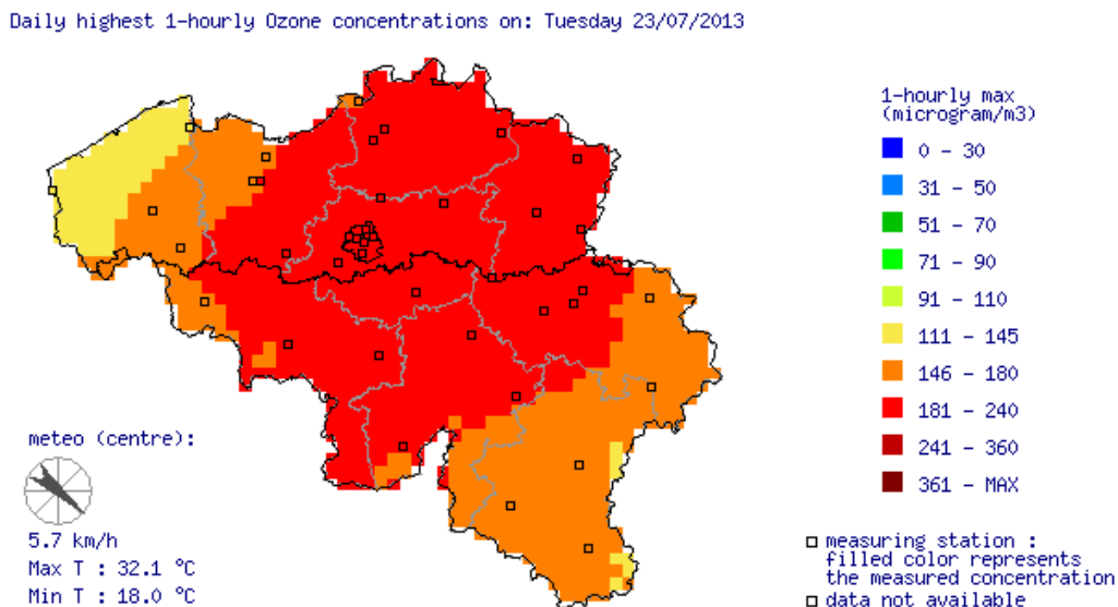
Figuur 6: Hoogste ozonconcentraties op 23 juli 2013.
