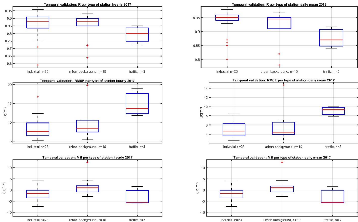
Figuur 21: temporele statistieken R, RMSE, MB (n=het aantal telemetrische stations) voor 2017 uurlijkse NO 2 -concentraties (links) NO 2 dagconcentraties (rechts)
