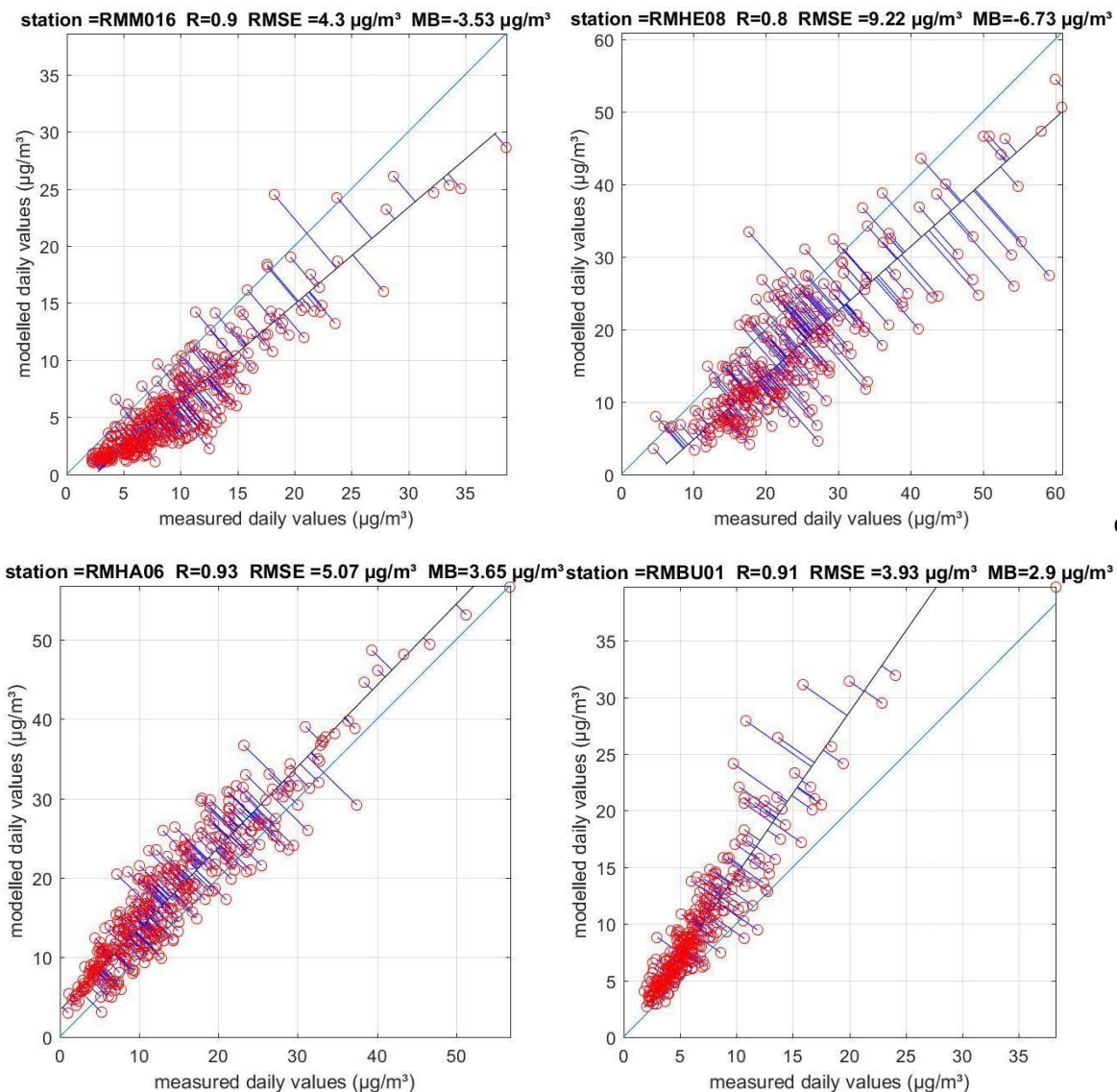
Figuur 30: Temporele validatie NO 2 daggemiddelde concentraties van de mobiele telemetrische stations in Wallonië voor 2017
