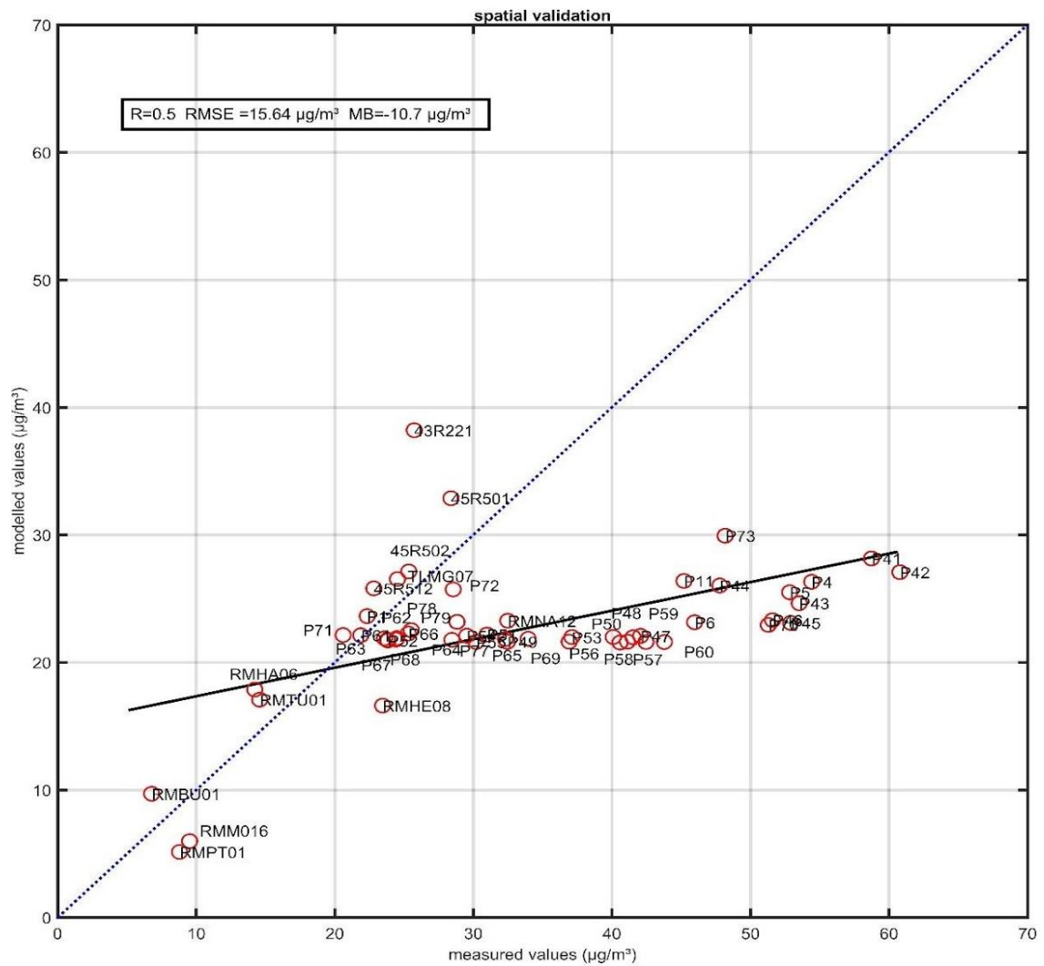
Figuur 10 : Ruimtelijke validatie RIO-IFDM NO 2 jaargemiddelden 2017 (alle beschikbare onafhankelijke metingen Wallonië: meetstations en passieve samplers).
