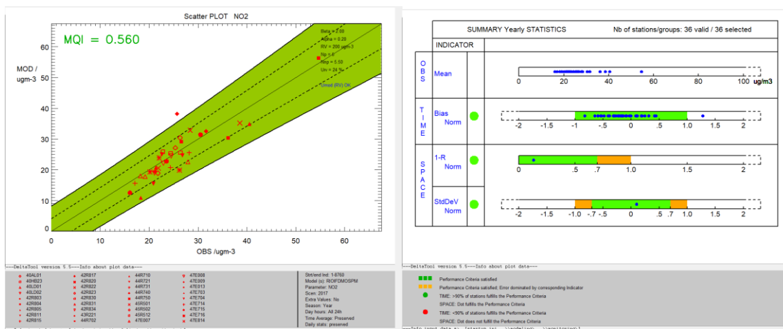
Figuur 36: DELTATOOL Model Quality Indicator en scatterplot NO2 jaargemiddelde (modelwaarden versus onafhankelijke metingen) onafhankelijke vaste telemetrische meetstations België RIO-IFDM 2017 (links) samenvattende statistieken (rechts)
