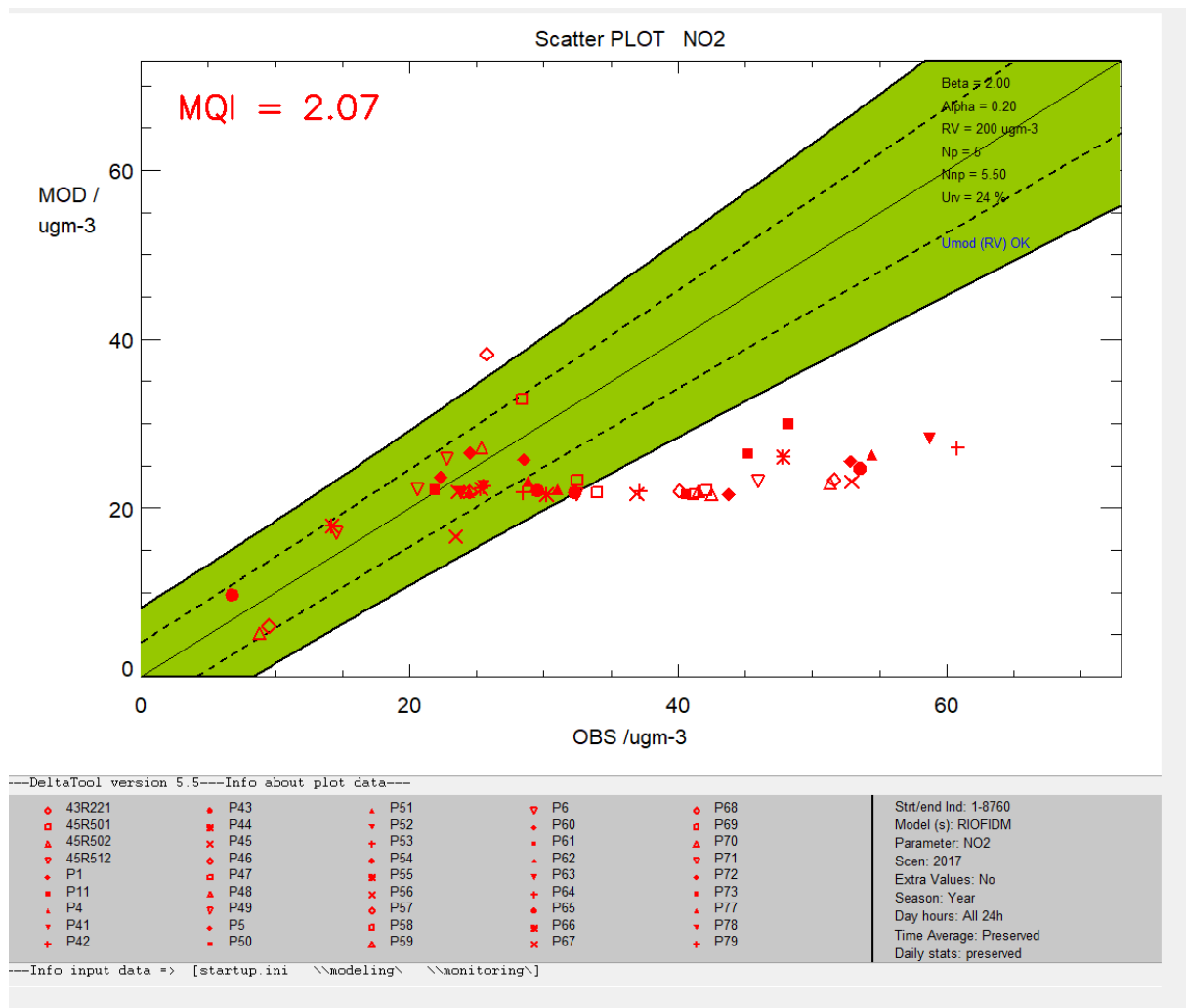
Figuur 11: DELTATOOL Model Quality Indicator en scatterplot NO 2 jaargemiddelde (modelwaarden versus onafhankelijke metingen) Wallonië RIO-IFDM 2017
