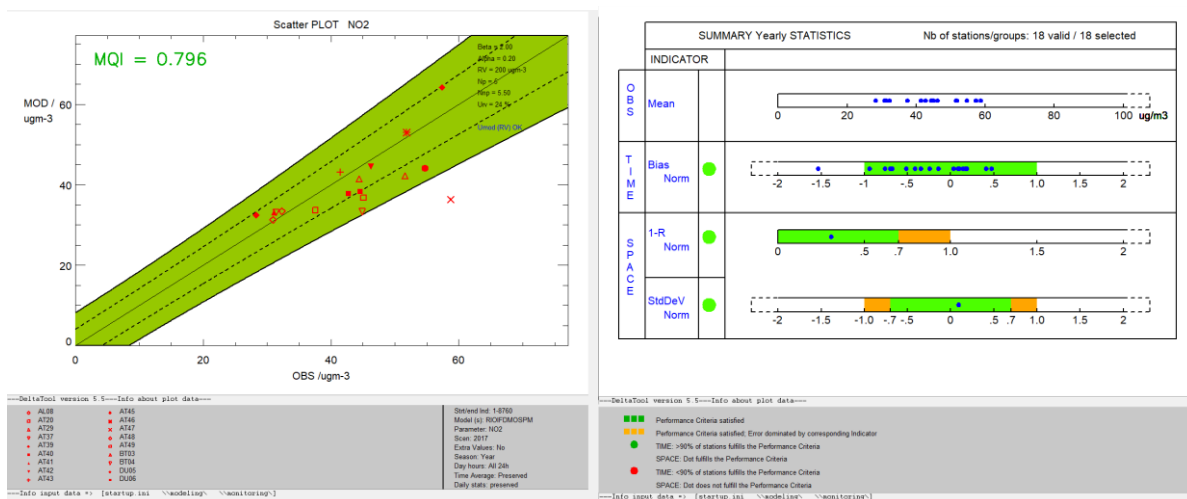
Figuur 33: DELTATOOL Model Quality Indicator en scatterplot NO2 jaargemiddelde (modelwaarden versus onafhankelijke vaste telemetrische metingen) passieve sampler meetcampagne Antwerpen ATMO-Street 2017 (links) en samenvattende statistieken (rechts)
