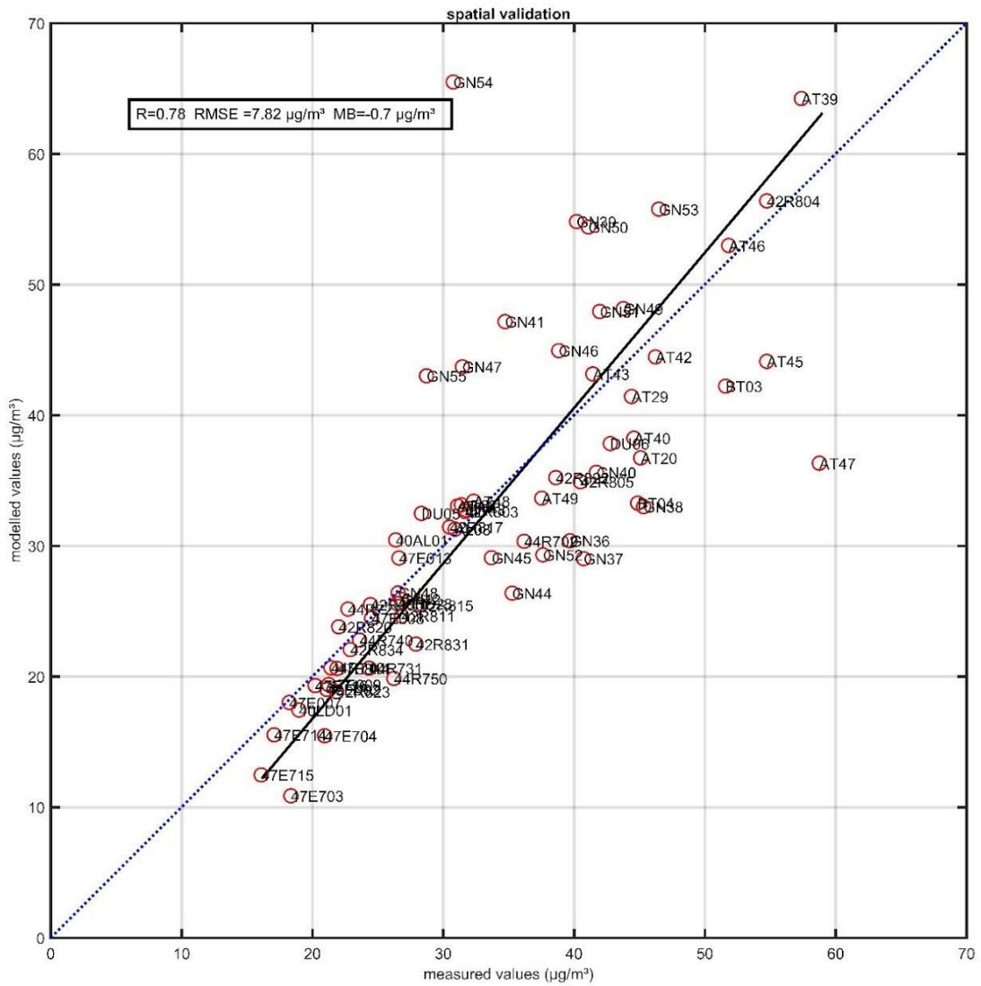
Figuur 8 : Ruimtelijke validatie ATMO-Street NO 2 jaargemiddelden 2017 (alle beschikbare onafhankelijke metingen Vlaanderen).
