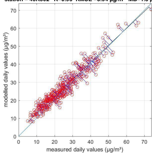
Figuur 23: Temporele validatie van de daggemiddelde \text{NO}_2 -concentraties stations 42R804 (verkeer), 42R805 (verkeer), 42R803 (stedelijke achtergrond) en 42R817 (stedelijke achtergrond) in Vlaanderen en 45R501 (stedelijke achtergrond) 45R502 (stedelijke achtergrond) in Wallonië voor 2017
