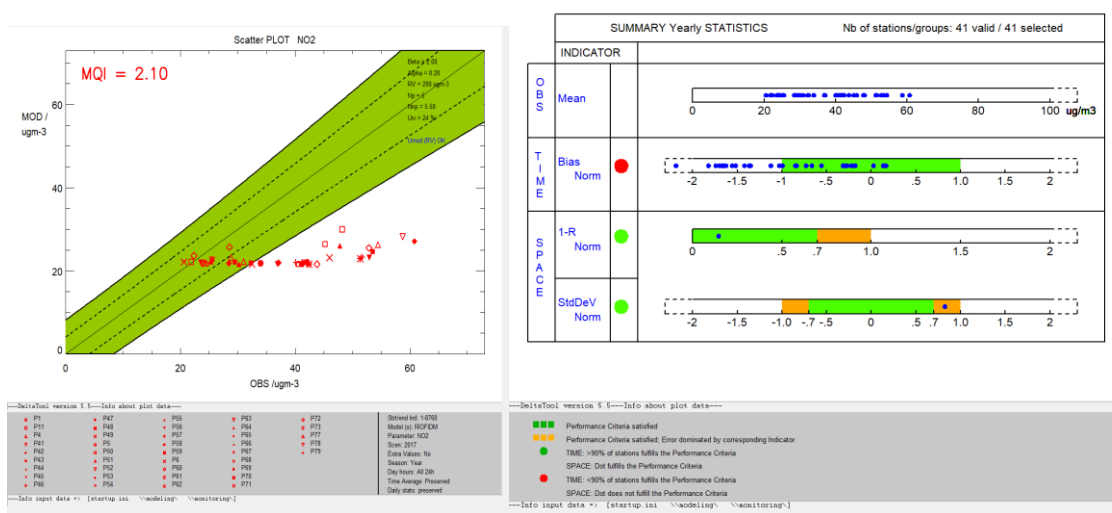
Figuur 35: DELTATOOL Model Quality Indicator en scatterplot NO2 jaargemiddelden (modelwaarden versus onafhankelijke metingen) passieve sampler meetcampagne Namen RIO-IFDM 2017 (links) samenvattende statistieken (rechts)
