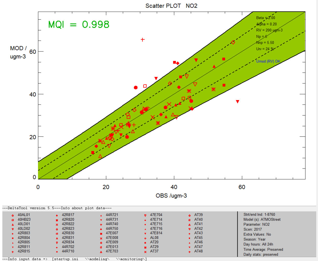
Figuur 9: DELTATOOL Model Quality Indicator en scatterplot NO2 jaargemiddelde (modelwaarden versus onafhankelijke metingen) Vlaanderen ATMO-Street 2017
