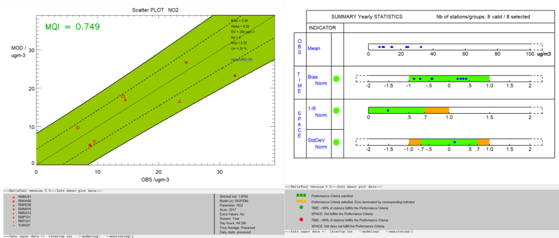
Figuur 37: DELTATOOL Model Quality Indicator en scatterplot NO2 jaargemiddelde (modelwaarden versus onafhankelijke metingen) onafhankelijke mobiele telemetrische meetstations Wallonië RIO-IFDM 2017 (links) samenvattende statistieken (rechts)
