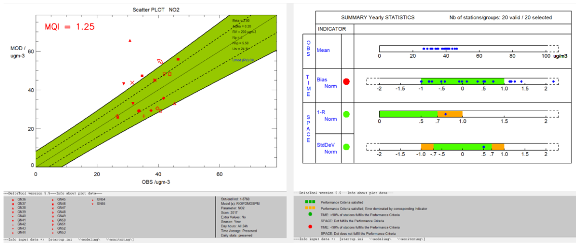
Figuur 34: DELTATOOL Model Quality Indicator en scatterplot NO2 jaargemiddelde (modelwaarden versus onafhankelijke vaste telemetrische metingen) passieve sampler meetcampagne Gent ATMO-Street 2017 (links) en samenvattende statistieken (rechts)
