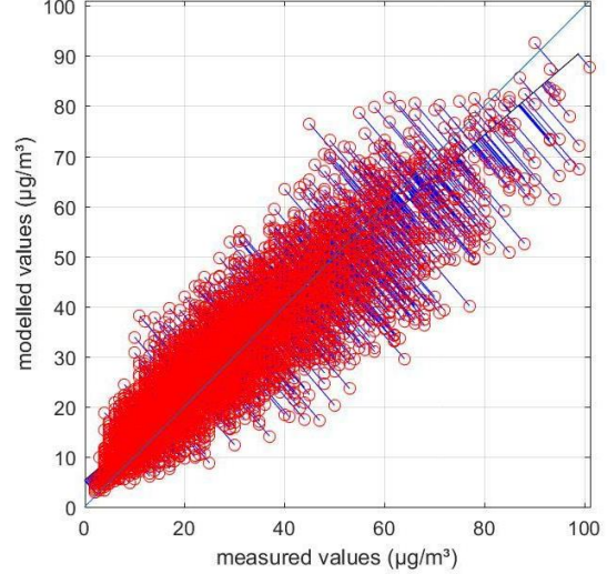
Figuur 22: Temporele validatie uurgemiddelde \text{NO}_2 -concentraties van de stations 42R804 (verkeer), 42R805 (verkeer), 42R803 (stedelijke achtergrond) en 42R817 (stedelijke achtergrond) in Vlaanderen en 45R501 (stedelijke achtergrond) 45R502 (stedelijke achtergrond) in Wallonië voor 2017
