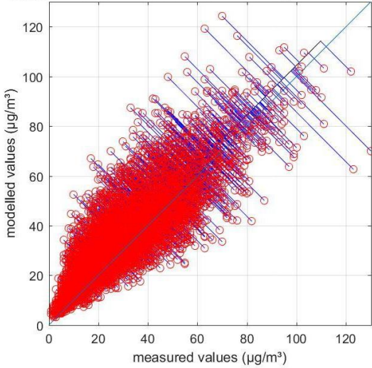
Figuur 22: Temporele validatie uurgemiddelde \text{NO}_2 -concentraties van de stations 42R804 (verkeer), 42R805 (verkeer), 42R803 (stedelijke achtergrond) en 42R817 (stedelijke achtergrond) in Vlaanderen en 45R501 (stedelijke achtergrond) 45R502 (stedelijke achtergrond) in Wallonië voor 2017
