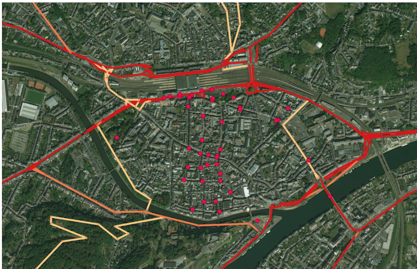
Figuur 18: Verkeersnetwerk gebruikt in Namen, en locatie van de passieve samplers.
