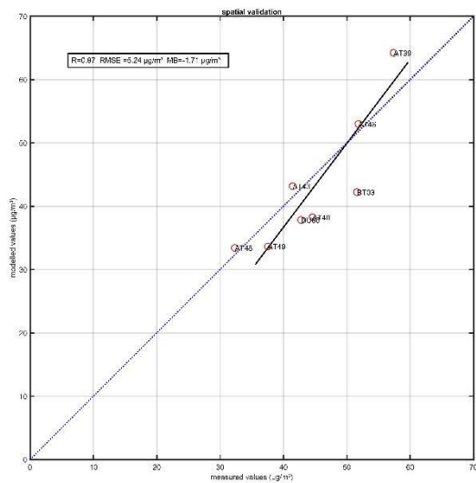
Figuur 13: Ruimtelijke validatie ATMO-Street jaargemiddelde NO 2 -concentratie 2017 passieve sampler meetcampagne Antwerpen met meetpunten waar streetcanyon effecten berekend zijn (links) en met meetpunten waar geen streetcanyon effecten berekend zijn (rechts)
