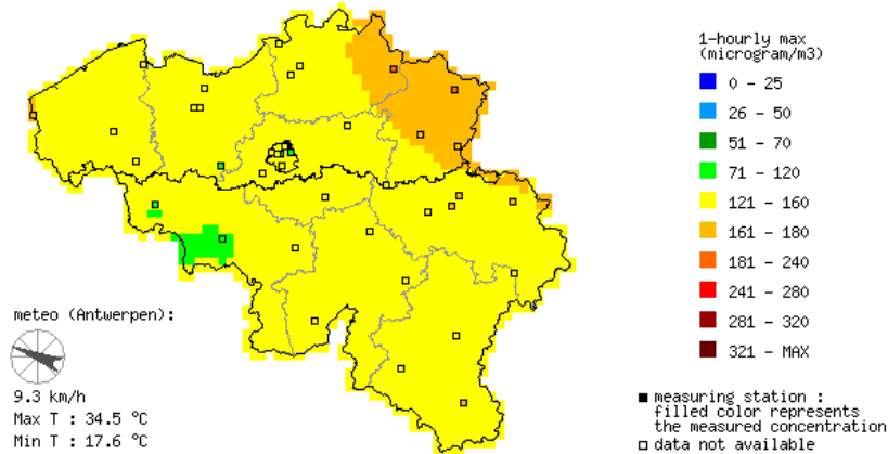
Concentrations horaires maximales pour le mardi 23 juillet 2019
