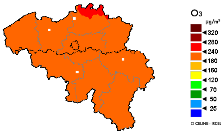
Concentrations horaires maximales prévues pour le 25 juillet 2019
