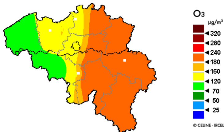
Concentrations horaires maximales prévues pour le jeudi 25 juillet
