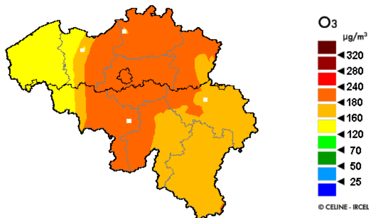
Concentrations horaires maximales prévues pour le mercredi 24 juillet 2019
