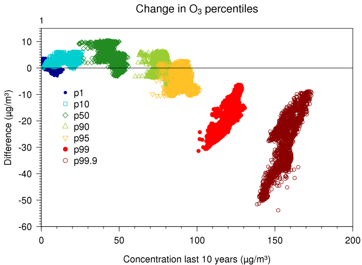
Figure 53 : évolution (différence entre les classes de concentrations) des centiles d'O 3 entre la période 1990-1999 et la période 2007-2016 en fonction des valeurs des centiles de la période 2007-2016 pour toutes les cellules de la grille RIO. Les données ont été générées sur base de la technique d'interpolation RIO. Les différentes couleurs indiquent les valeurs des centiles (cf. légende).
