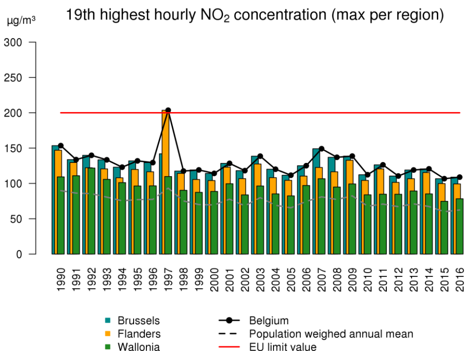
Figure 35 : évolution du maximum de la 19 ème valeur horaire la plus élevée de NO 2 dans les trois Régions et en Belgique, calculée sur base de la technique d'interpolation RIO.
