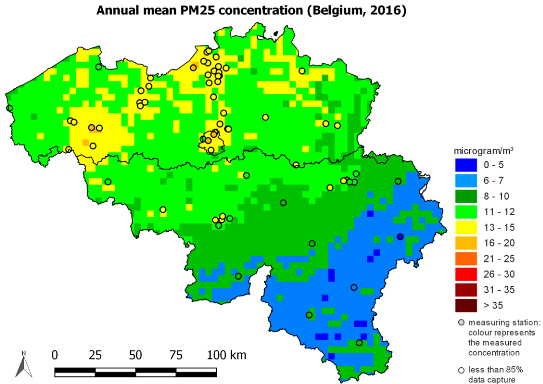
Figure 19: distribution spatiale de la concentration moyenne annuelle de \text{PM}_{2,5} en Belgique en 2016. Toutes les données ont été calculées sur base de la technique d'interpolation RIO.
