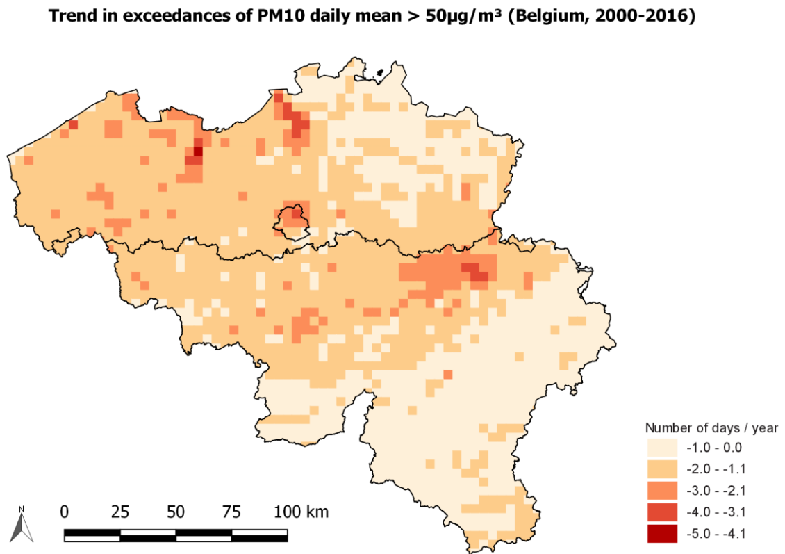
Figure 15: distribution spatiale de la tendance du nombre de jours de moyenne journalière > 50 µg/m 3 sur la période 2000-2016 (nombre de jours/an). Toutes les données ont été calculées sur base de la technique d'interpolation RIO.
