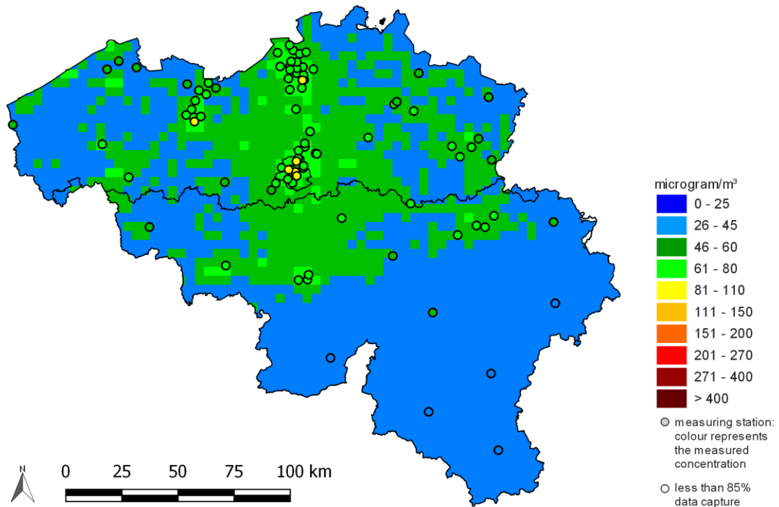
Figure 33: distribution spatiale de la 19 ème concentration moyenne horaire de NO 2 la plus élevée en Belgique en 2016 Toutes les données ont été calculées sur base de la technique d'interpolation RIO.
