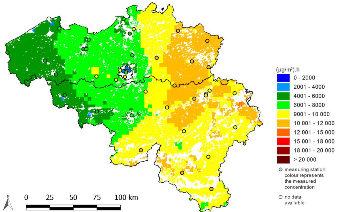
Figure 44: distribution spatiale de la surcharge pour la végétation (AOT40 végétation), en moyenne sur 5 ans pour 2012-2016. «No data available» signifie que les données ne respectent pas les critères établis dans l'annexe VII de la directive 2008/50/CE pour l'agrégation des données de mesure. Toutes les données ont été calculées sur base de la technique d'interpolation RIO.
