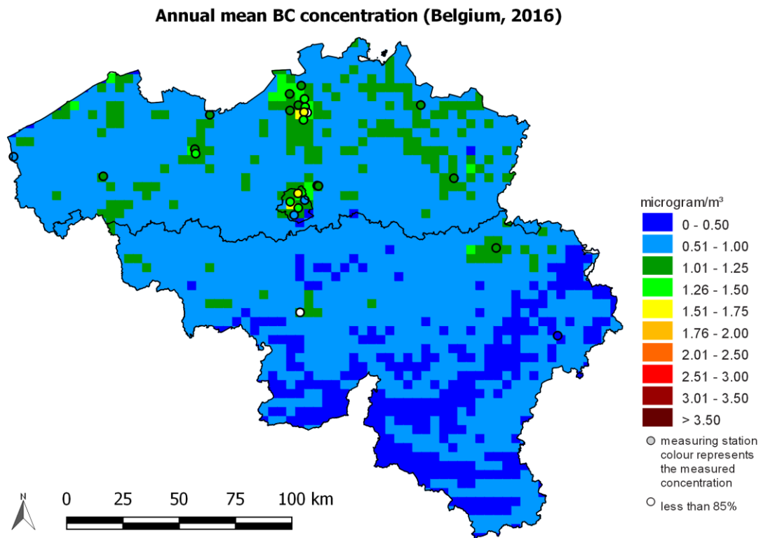
Figure 25: distribution spatiale de la concentration moyenne annuelle de BC en Belgique en 2016. Toutes les données ont été calculées sur base de la technique d'interpolation RIO.
