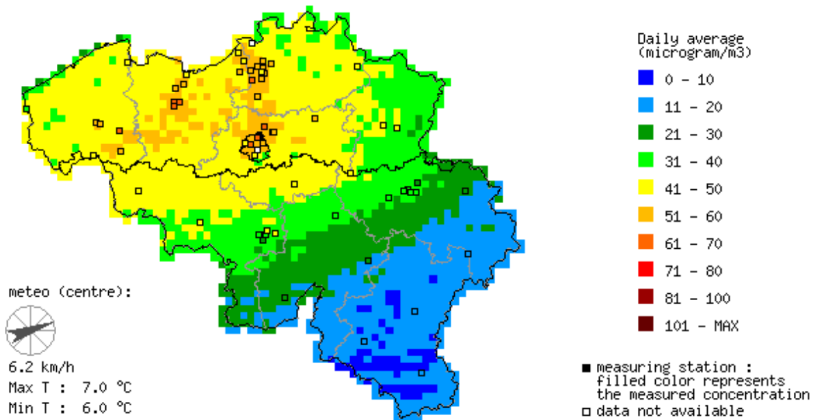
Figure 4: Moyenne journalière des concentrations de particules fines pour la journée du 18 décembre 2016.
