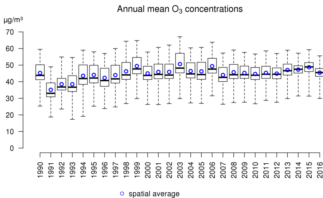
Figure 50: diagramme en boîtes des concentrations moyennes d'O 3 sur la période 1990-2016. La moyenne spatiale est indiquée par les cercles bleus. Toutes les données ont été calculées sur base de la technique d'interpolation RIO.
