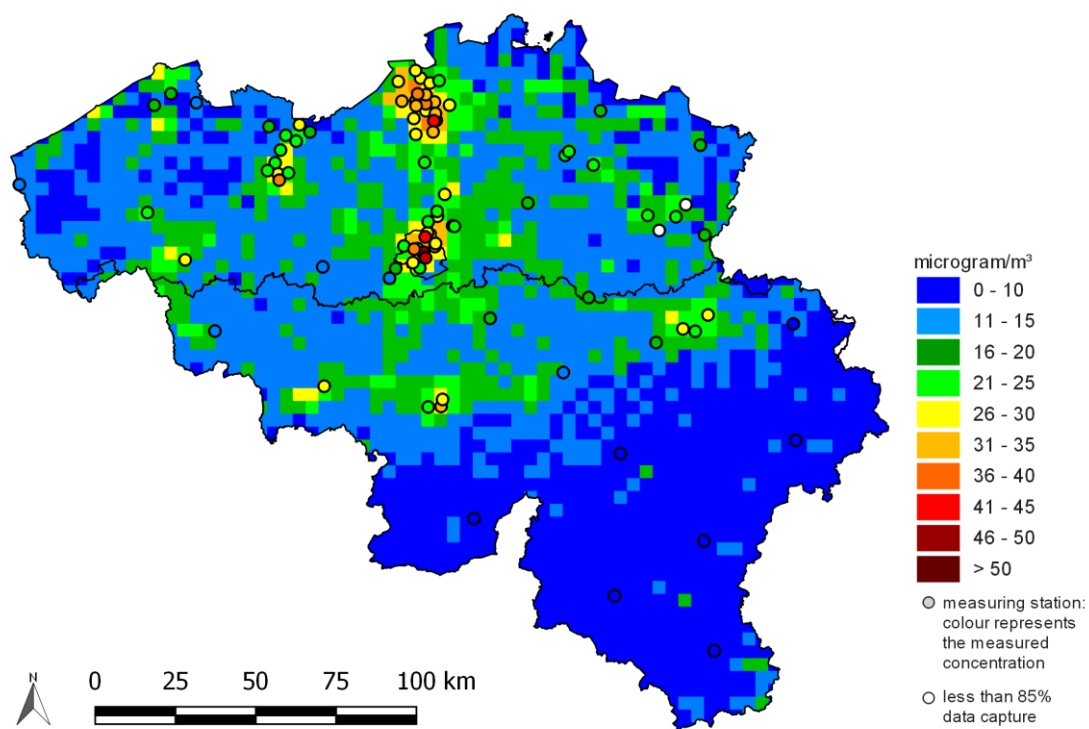
Figure 27: distribution spatiale de la concentration moyenne annuelle de NO 2 en Belgique en 2016. Toutes les données ont été calculées sur base de la technique d'interpolation RIO.
