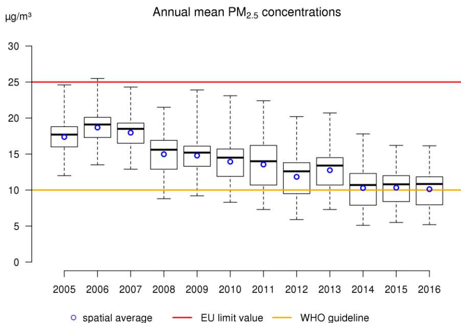
Figure 20 : diagramme en boîtes des concentrations moyennes annuelles de PM_{2.5} ( \mu g/m^3 ) sur la période 2005-2016. La moyenne spatiale est indiquée par les cercles bleus. Toutes les données ont été calculées sur base de la technique d'interpolation RIO.
