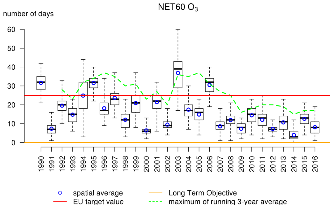
Figure 39: Diagramme en boîtes du nombre de jours caractérisés par un maximum journalier des concentrations d’ozone en moyennes sur 8 heures > 120 µg/m 3 en Belgique durant la période 1990-2016. La moyenne spatiale est indiquée par les cercles bleus. La ligne pointillée verte donne le maximum du nombre de dépassements moyenné sur 3 ans en Belgique. Toutes les données ont été calculées sur base de la technique d’interpolation RIO.
