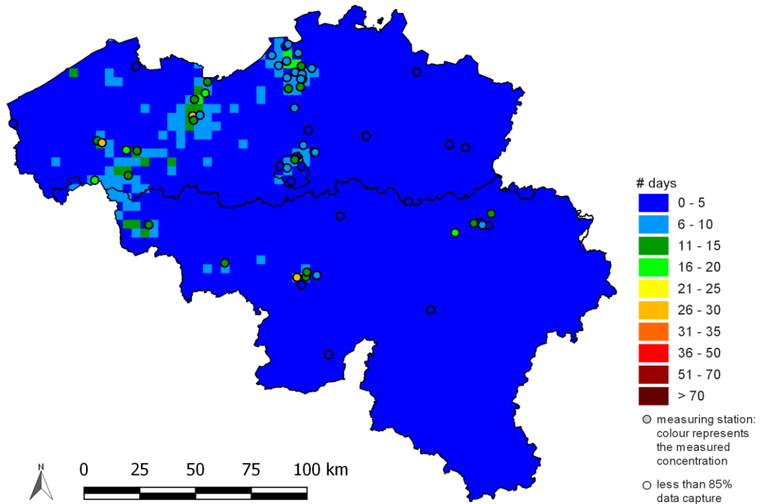
Figure 12: distribution spatiale du nombre de jours en 2016 où la concentration moyenne journalière de PM 10 a dépassé 50 µg/m 3 en Belgique. Toutes les données ont été calculées sur base de la technique d'interpolation RIO.
