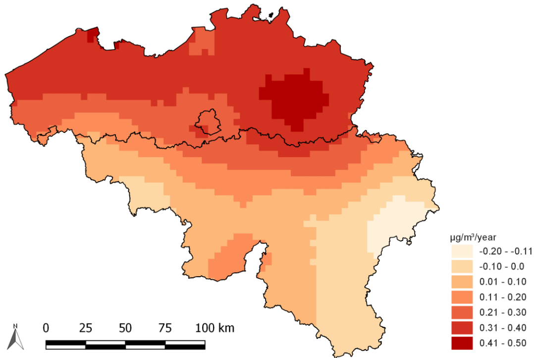
Figure 52: distribution spatiale de la tendance de la concentration moyenne annuelle d'O 3 (µg/m 3 /an) sur la période 1990-2016. Les données utilisées pour l'analyse de tendance ont été générées sur base de la technique d'interpolation RIO.
