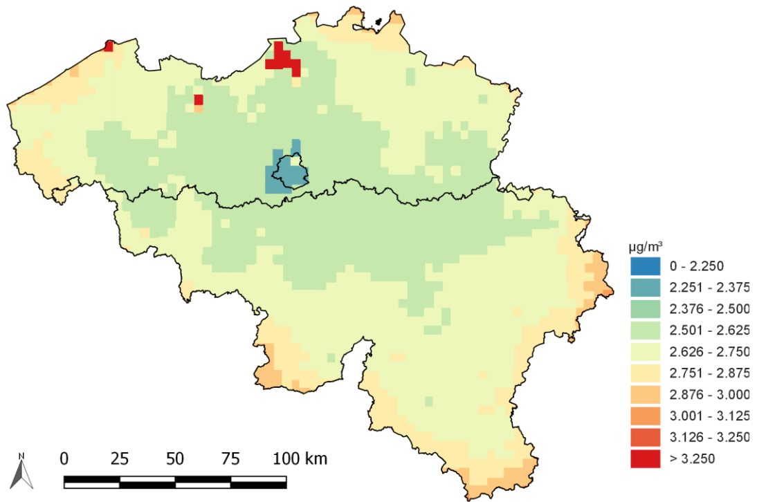
Distribution spatiale de l'erreur absolue (µg/m 3 ) pour la concentration moyenne annuelle de O 3 .
