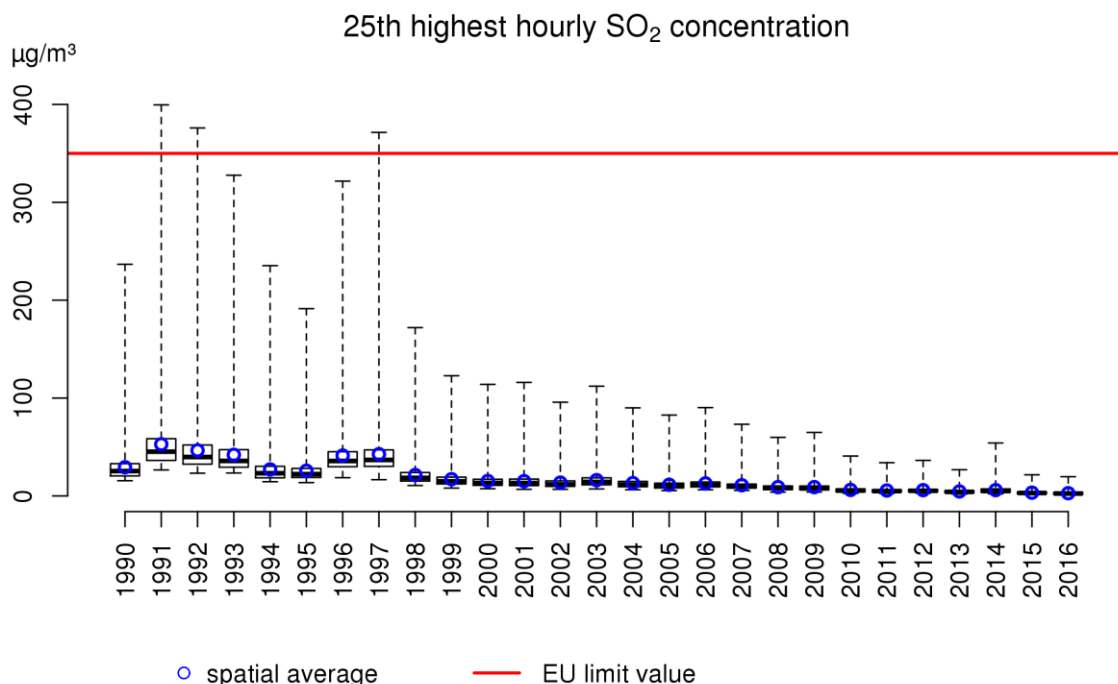
Figure 57: diagramme en boîtes de la 25 ème concentration moyenne horaire de SO 2 la plus élevée sur la période 1990-2016 en Belgique sur base de la technique d'interpolation RIO.
