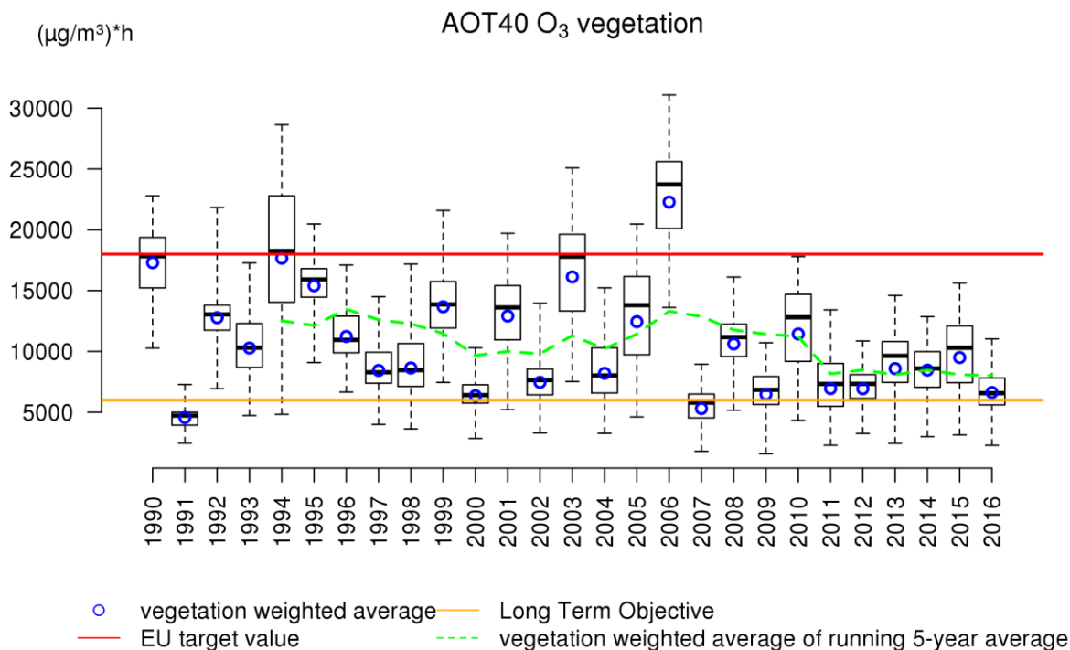
Figure 45: diagramme en boîtes de la surcharge pour la végétation (AOT40) en Belgique (1990-2016). Les moyennes pondérées en fonction de la végétation pour la Belgique sont représentées par les cercles bleus. La ligne pointillée verte indique la moyenne pondérée en fonction de la végétation de l'AOT40 sur 5 ans. Toutes les données ont été calculées sur base de la technique d'interpolation RIO.
