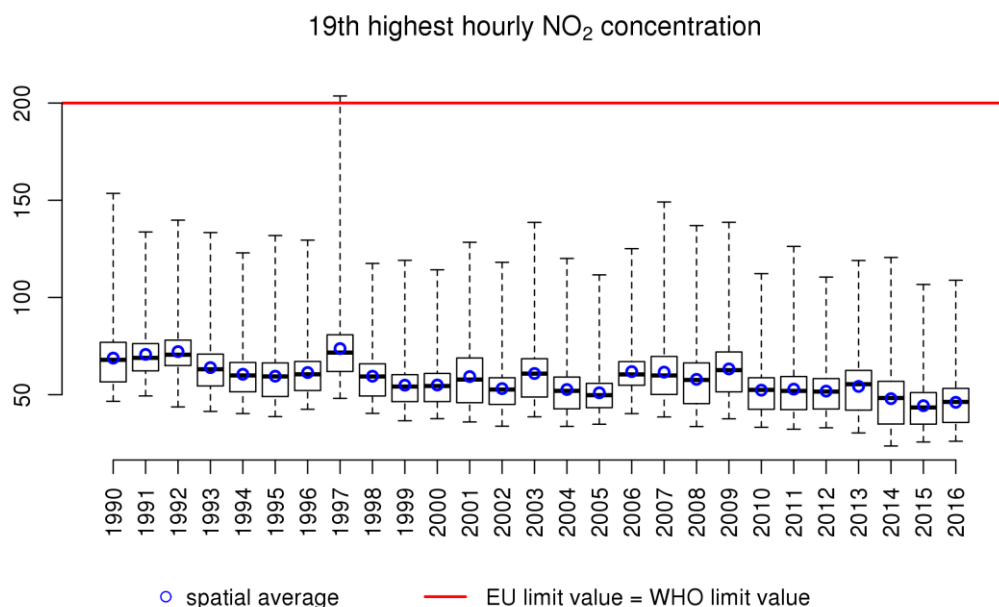
Figure 34: diagramme en boîtes de la 19 ème concentration horaire moyenne la plus élevée de NO 2 (µg/m 3 ) sur la période 1990-2016. La moyenne spatiale est indiquée par les cercles bleus. Toutes les données ont été calculées sur base de la technique d'interpolation RIO.
