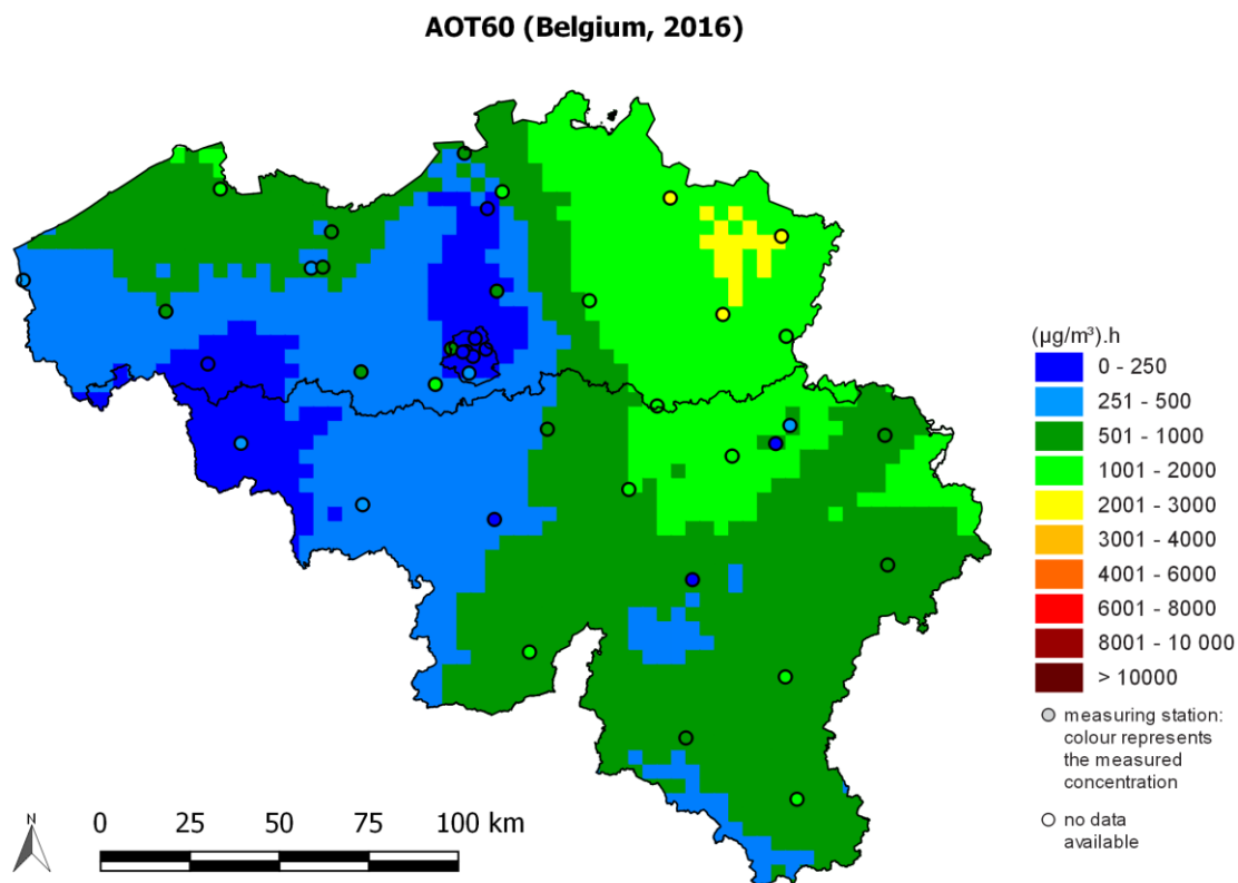
Figure 42: distribution spatiale de la surcharge d’ozone (AOT60) en 2016. «No data» signifie que les données ne respectent pas les critères établis dans l’annexe VII de la 2008/50/CE pour l’agrégation des données de mesure. Toutes les données ont été calculées sur base de la technique d’interpolation RIO.
