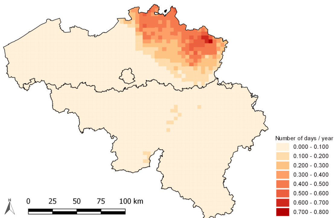
Figure 40: tendance (nombre de jours / an) du nombre de jours pour lesquels le maximum journalier de la concentration moyenne sur 8 heures d’ozone est supérieure à 120 µg/m 3 (NET60) durant la période 1990-2016. Toutes les données ont été calculées sur base de la technique d’interpolation RIO.
