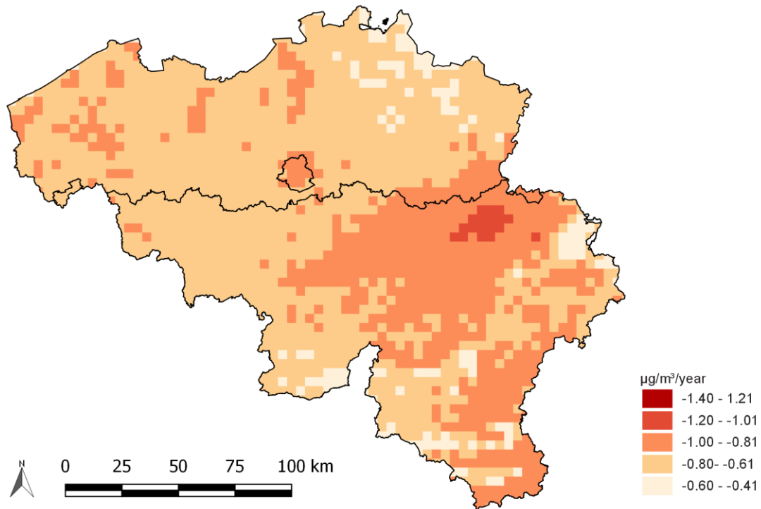
Figure 10: distribution spatiale de la tendance temporelle des concentrations moyennes annuelles de PM10 ( \mu\text{g}/\text{m}^3/\text{an} ). Toutes les données ont été calculées sur base de la technique d'interpolation RIO.
