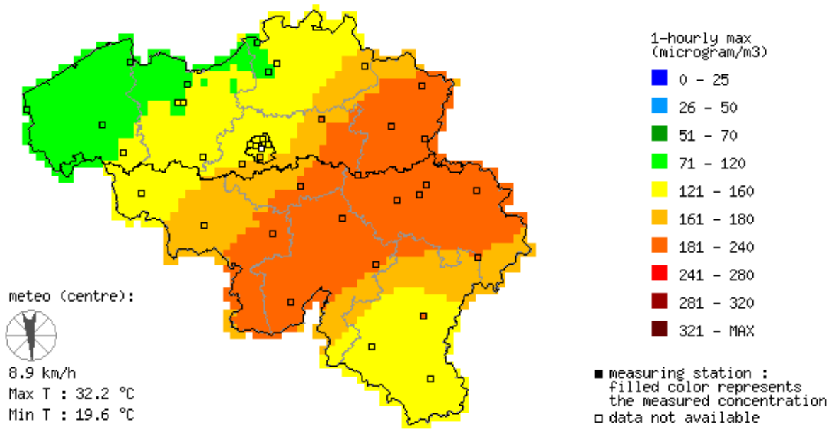
Figure 5: Concentrations d’ozone horaires maximales du 26 août 2016.
