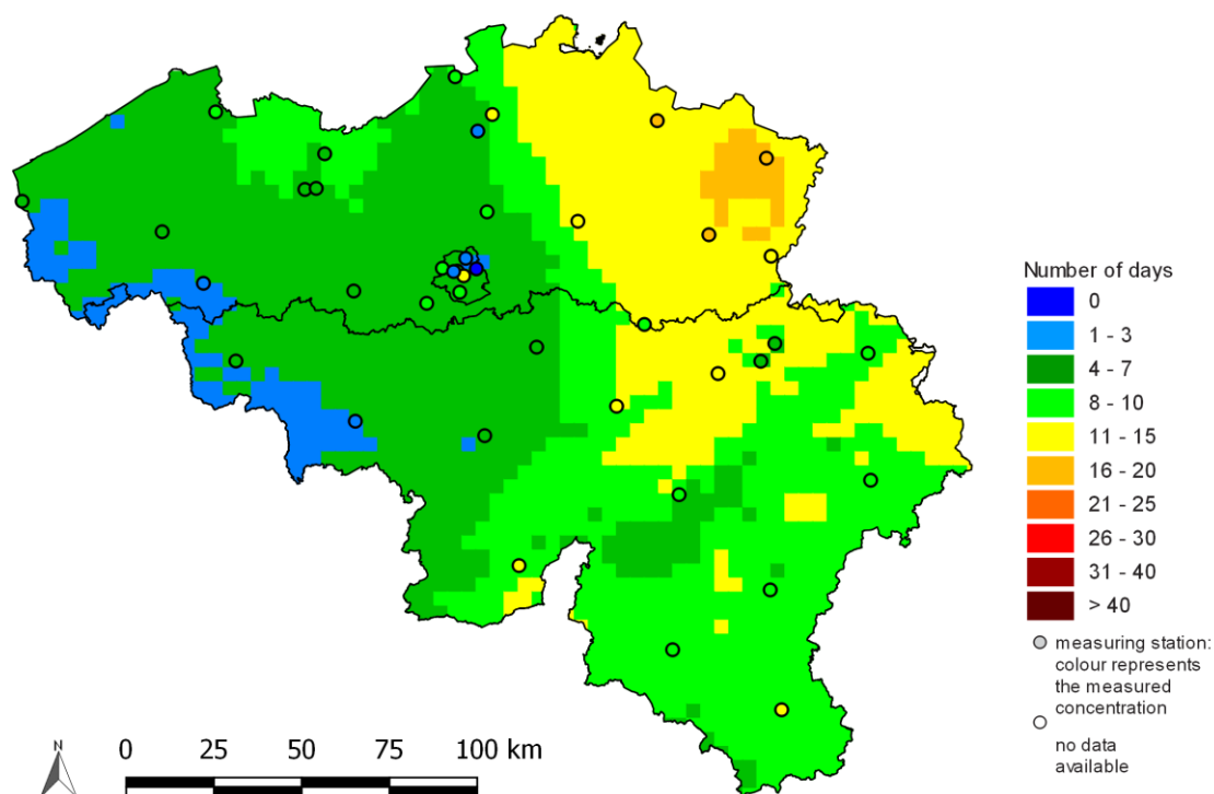
Figure 38: distribution spatiale du NET60 en moyenne sur 2014, 2015 et 2016. « No data available » signifie que les données ne respectent pas les critères établis dans l'annexe VII de la directive 2008/50/CE pour l'agrégation des données de mesure. Toutes les données ont été calculées sur base de la technique d'interpolation RIO.
