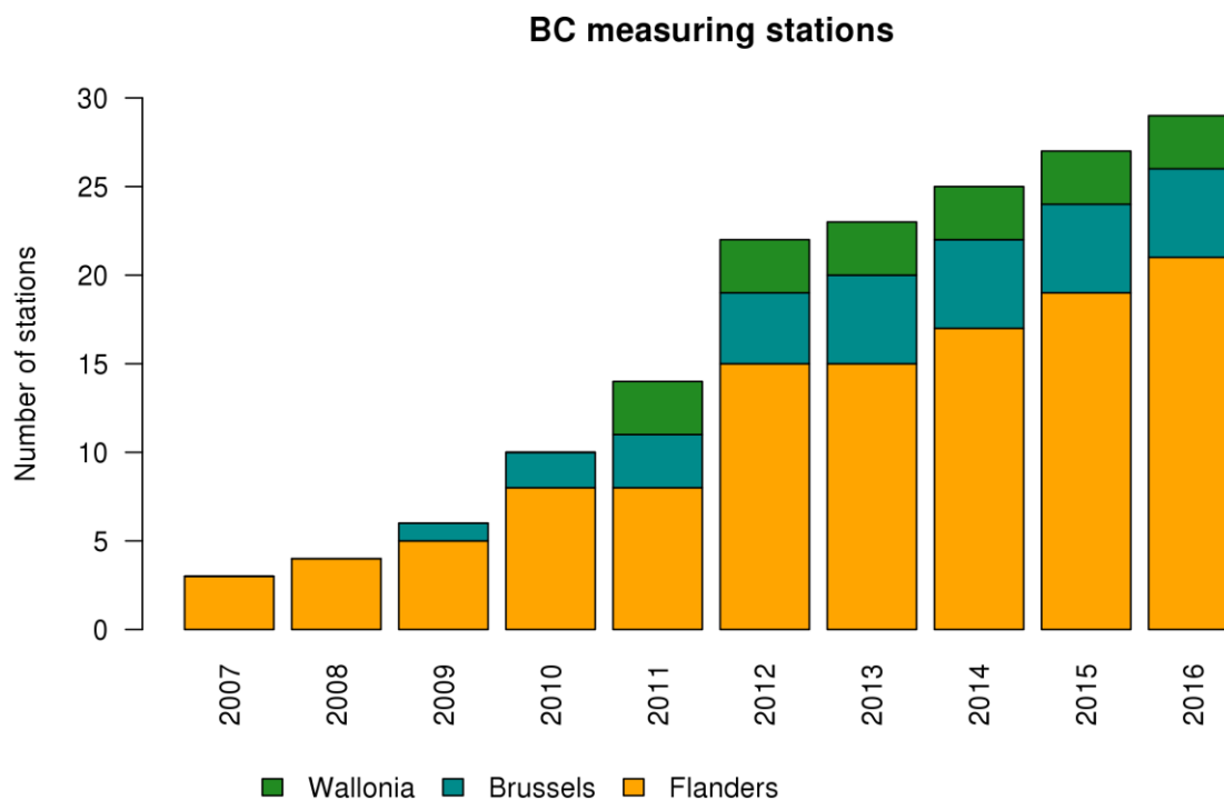
Figure 24: évolution du nombre de stations de mesure du BC en Belgique.
