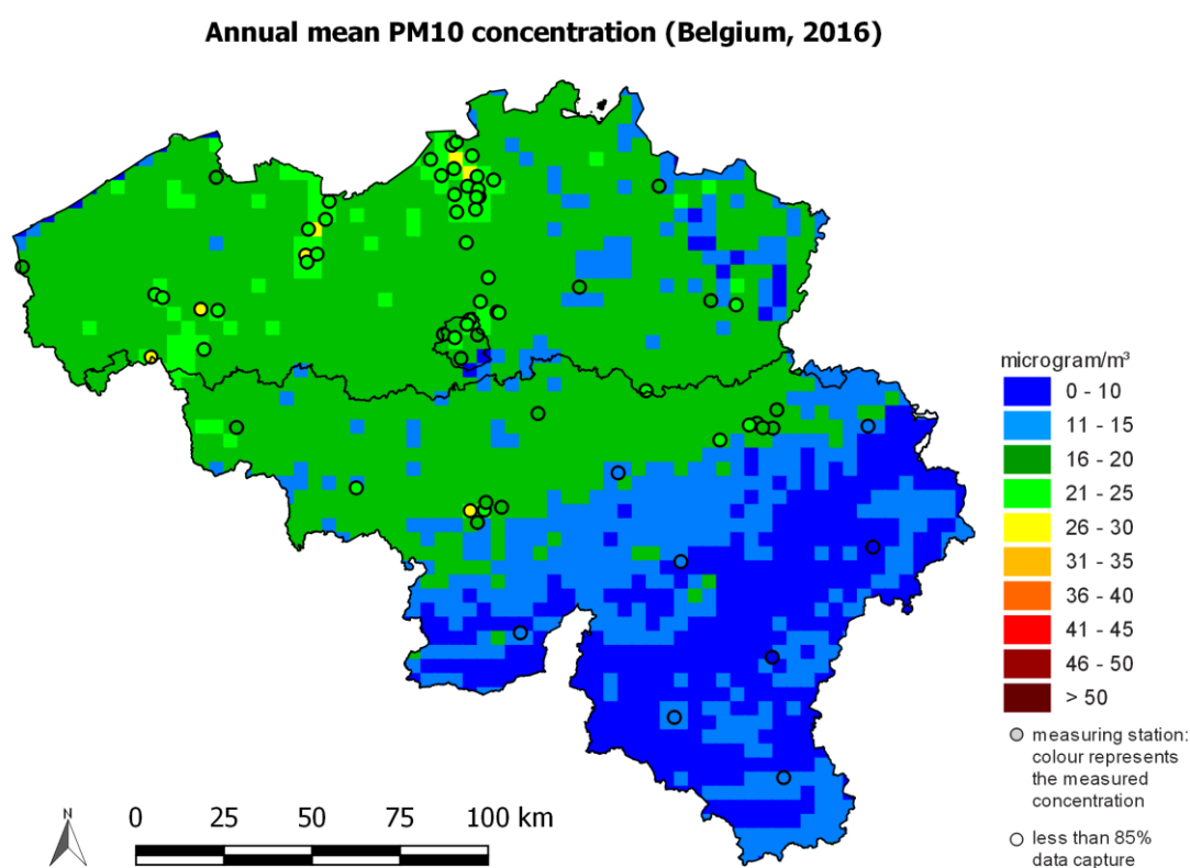
Figure 7: distribution spatiale de la concentration moyenne annuelle de PM 10 en Belgique en 2016. Toutes les données ont été calculées sur base de la technique d'interpolation RIO.
