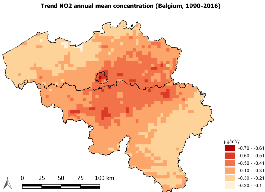
Figure 31: tendance (µg/m 3 /an) des concentrations moyennes annuelles de NO 2 au cours de la période 1990-2016. Toutes les données ont été calculées sur base de la technique d'interpolation RIO.
