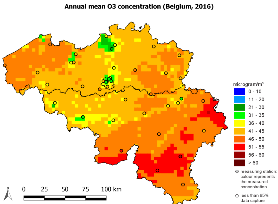
Figure 48: distribution spatiale de la concentration moyenne annuelle de O 3 en Belgique en 2016. Toutes les données ont été calculées sur base de la technique d'interpolation RIO.
