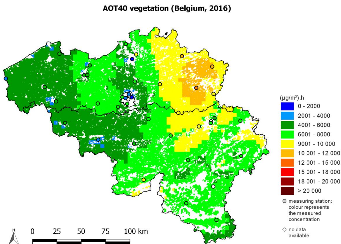
Figure 43: distribution spatiale de la surcharge pour la végétation (AOT40_végétation), 2016. « No data available » signifie que les données ne respectent pas les critères établis dans l'annexe VII de la directive 2008/50/CE pour l'agrégation des données de mesure. Toutes les données ont été calculées sur base de la technique d'interpolation RIO.
