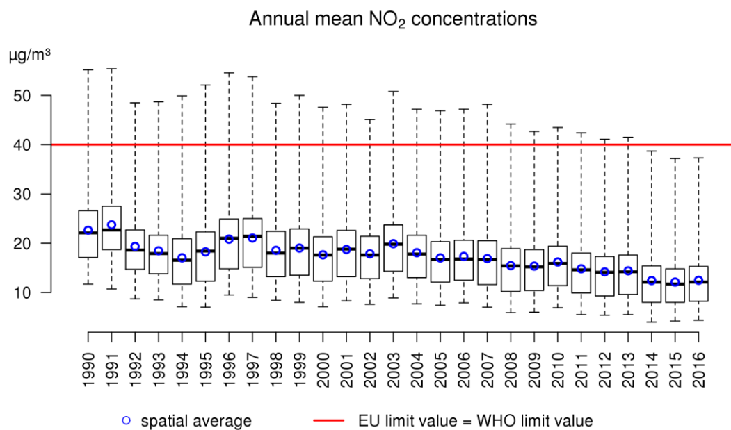
Figure 29: diagramme en boîtes des concentrations moyennes annuelles de NO 2 (µg/m 3 ) sur la période 1990-2016 en Belgique. La moyenne spatiale est indiquée par les cercles bleus. Toutes les données ont été calculées sur base de la technique d'interpolation RIO.
