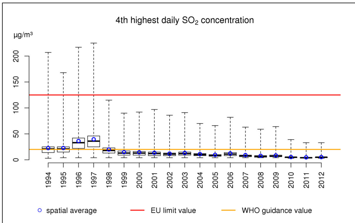
Figure 57: diagramme en boîtes de la 4 ème concentration moyenne horaire de SO 2 la plus élevée sur la période 1994-2012 en Belgique sur base de la technique d'interpolation RIO.
