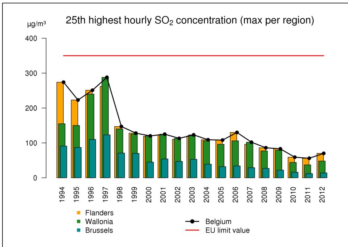
Figure 54 : évolution de la 25 ème concentration moyenne horaire de SO 2 maximale par Région et en Belgique sur base de la technique d'interpolation RIO.
