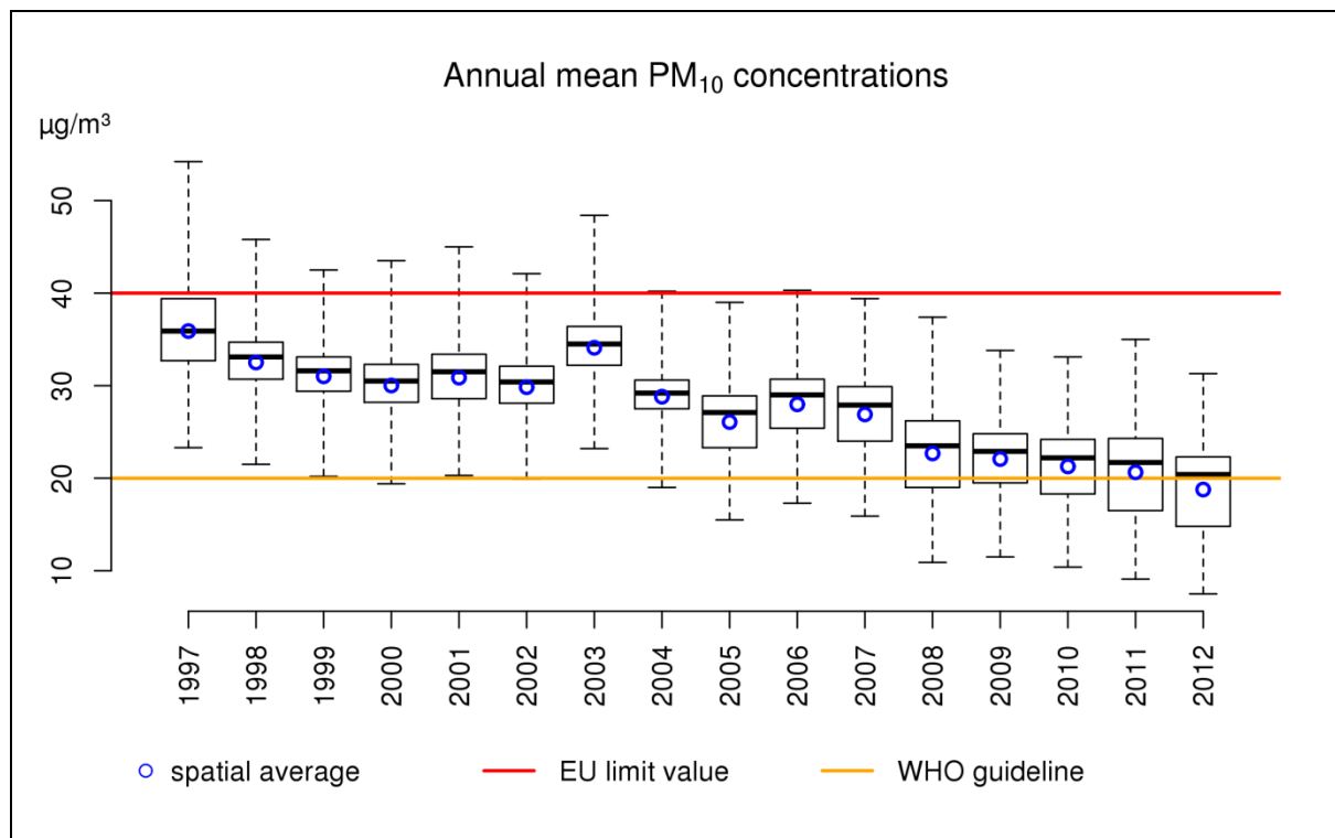
Figure 9: diagramme en boîtes des concentrations moyennes annuelles de PM_{10} ( \mu\text{g}/\text{m}^3 ) sur la période 1997-2012 en Belgique. La moyenne spatiale est indiquée par les cercles bleus. Toutes les données ont été calculées sur base de la technique d'interpolation RIO.
