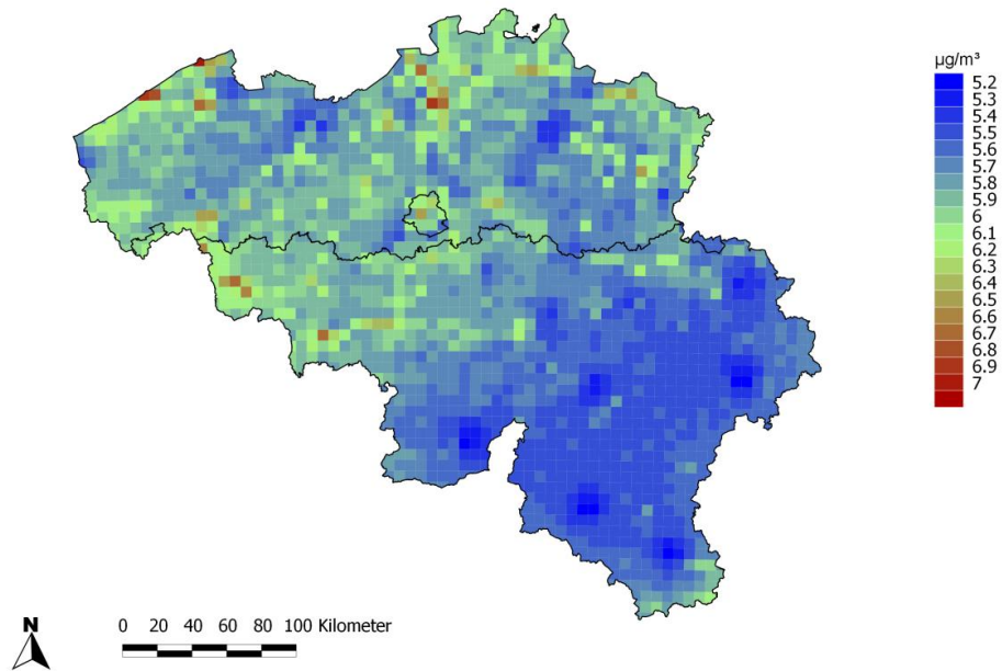
Distribution spatiale de l'erreur absolue ( \mu\text{g}/\text{m}^3 ) pour la concentration moyenne annuelle de NO 2 .
