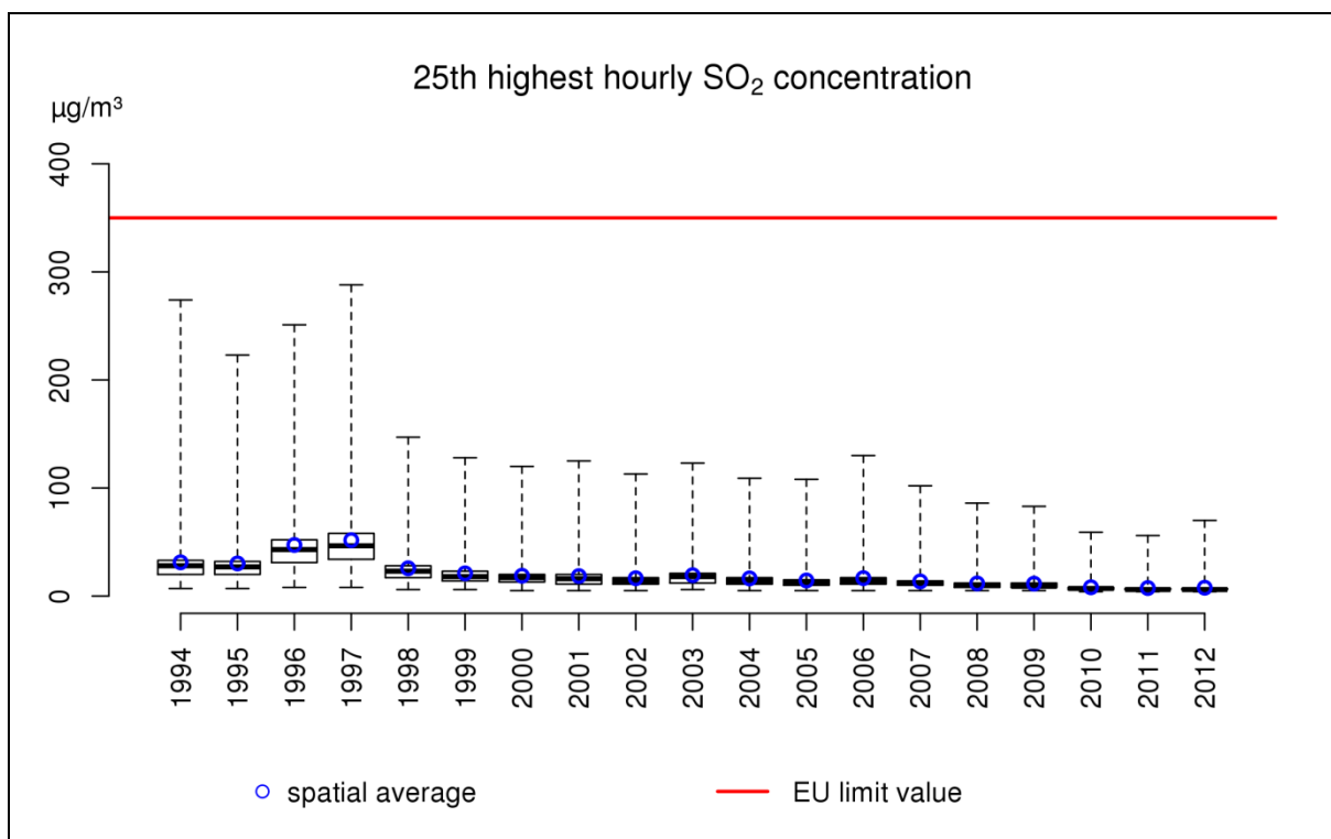
Figure 55: diagramme en boîtes de la 25 ème concentration moyenne horaire de SO 2 la plus élevée sur la période 1994-2012 en Belgique sur base de la technique d'interpolation RIO.
