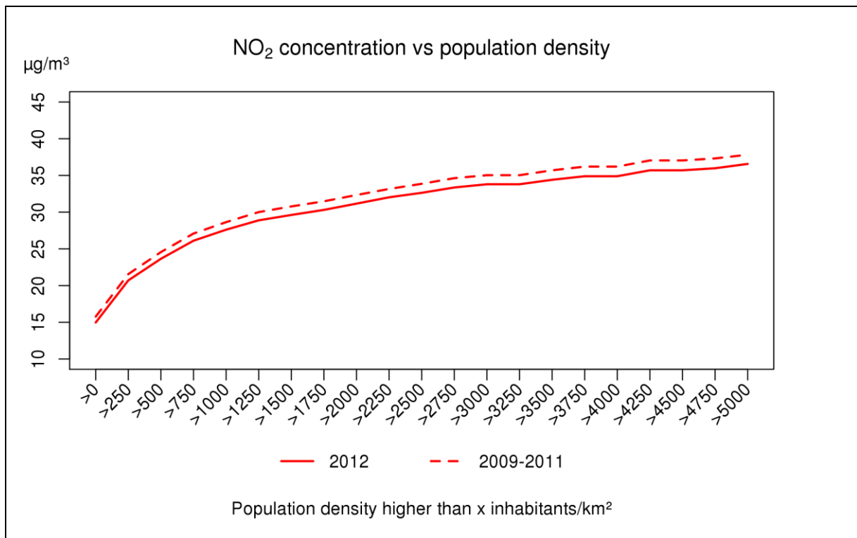
Figure 27: relations entre les concentrations moyennes annuelles interpolées de NO 2 et la densité de population (habitants/km 2 ). Toutes les données ont été calculées sur base de la technique d'interpolation RIO.
