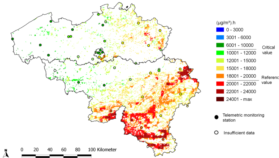
Figure 46: distribution spatiale de la surcharge d’ozone pour les forêts (AOT40_forêts), en moyenne sur 5 ans pour les années 2008-2012 . « Insufficient data » signifie que les données ne respectent pas les critères établis dans l’annexe VII de la 2008/50/CE pour l’agrégation des données de mesure. Toutes les données ont été calculées sur base de la technique d’interpolation RIO.
