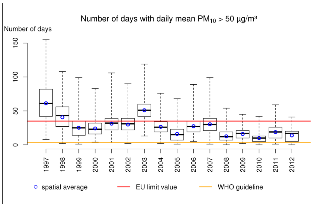
Figure 15: évolution du nombre maximum de jours par an où la concentration moyenne journalière de PM 10 était supérieure à 50 µg/m 3 en Belgique et dans les trois Régions. Toutes les données ont été calculées sur base de la technique d'interpolation RIO.
