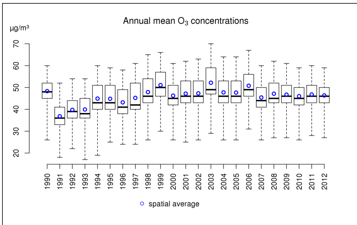
Figure 49: diagramme en boîtes des concentrations moyennes d'O 3 sur la période 1990-2012. La moyenne spatiale est indiquée par les cercles bleus. Toutes les données ont été calculées sur base de la technique d'interpolation RIO.
