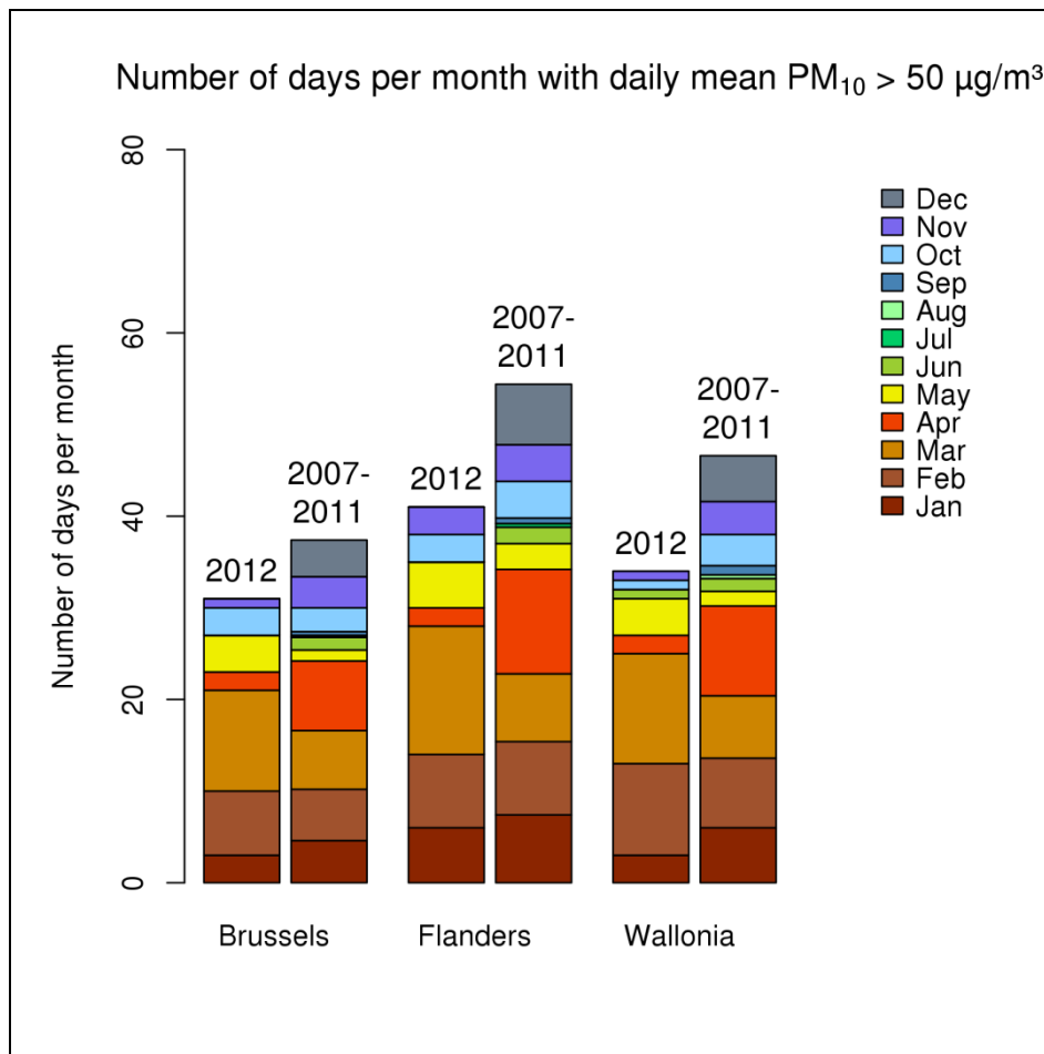
Figure 18: nombre maximal de jours par mois où la norme moyenne journalière de 50 \mu\text{g}/\text{m}^3 a été dépassée localement en Régions bruxelloise, flamande et wallonne en 2012, et au cours des cinq années précédentes. Toutes les données ont été calculées sur base de la technique d'interpolation RIO.
