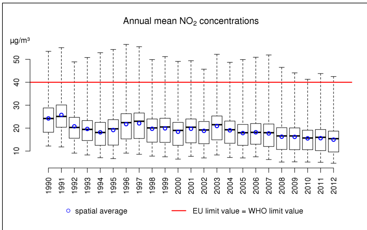
Figure 28: diagramme en boîtes des concentrations moyennes annuelles de NO 2 (µg/m 3 ) sur la période 1990-2012 en Belgique. La moyenne spatiale est indiquée par les cercles bleus. Toutes les données ont été calculées sur base de la technique d'interpolation RIO.
