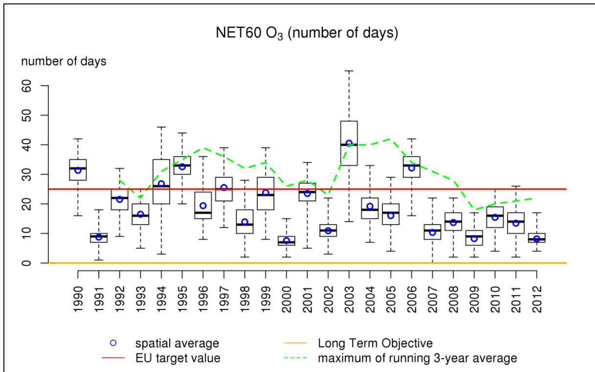
Figure 38: diagramme en boîtes du nombre de jours caractérisés par un maximum journalier des concentrations d’ozone en moyennes sur 8 heures > 120 µg/m 3 en Belgique durant la période 1990-2012. La moyenne spatiale est indiquée par les cercles bleus. La ligne pointillée verte donne le maximum du nombre de dépassements moyenné sur 3 ans en Belgique. Toutes les données ont été calculées sur base de la technique d’interpolation RIO.
