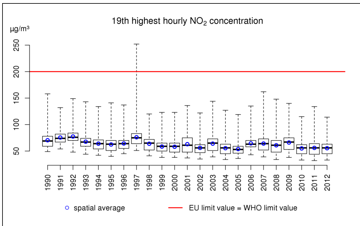
Figure 33: diagramme en boîtes de la 19 ème concentration horaire moyenne la plus élevée de NO 2 (µg/m 3 ) sur la période 1990-2012. La moyenne spatiale est indiquée par les cercles bleus. Toutes les données ont été calculées sur base de la technique d'interpolation RIO.
