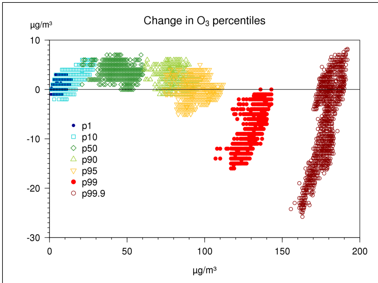
Figure 52 : évolution (différence entre les classes de concentrations) des centiles d'O 3 entre la période 1990-2001 et la période 2002-2012 en fonction des valeurs des centiles de la période 2002-2012 pour toutes les cellules de la grille RIO. Les données ont été générées sur base de la technique d'interpolation RIO. Les différentes couleurs indiquent les valeurs des centiles (cf. légende).
