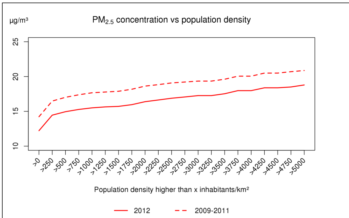
Figure 24: Relations entre les concentrations moyennes annuelles interpolées de PM_{2.5} et la densité de population (nombre d'habitants/ km^2 ) supérieure à un seuil donné (précisé sur l'axe horizontal du graphique). Toutes les données ont été calculées sur base de la technique d'interpolation RIO.
