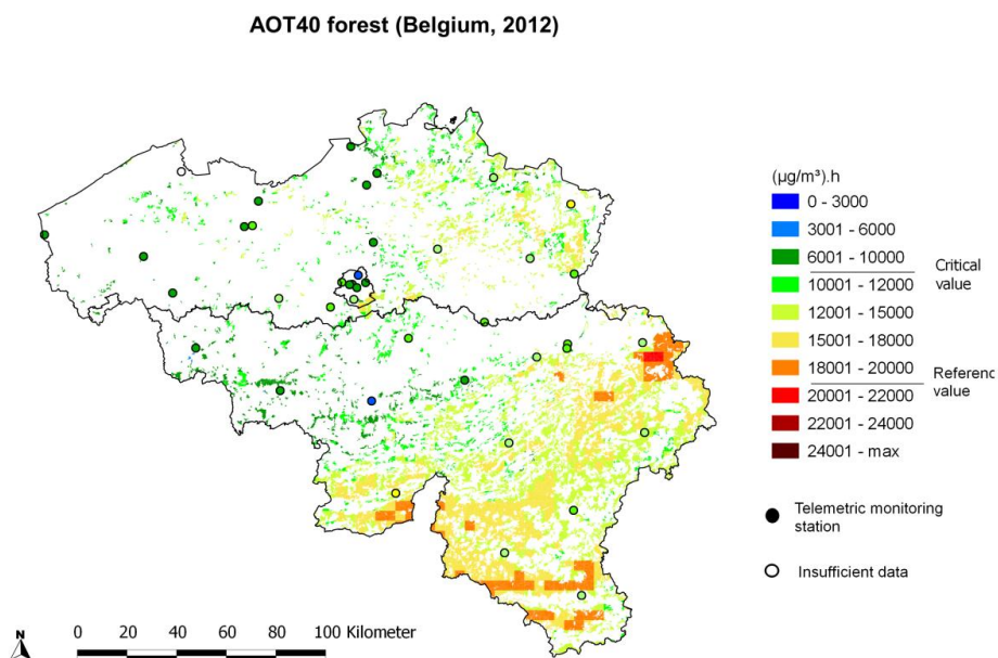
Figure 45: distribution spatiale de la surcharge de zone pour les forêts (AOT40_forêts) en 2012 . « Insufficient data » signifie que les données ne respectent pas les critères établis dans l'annexe VII de la 2008/50/CE pour l'agrégation des données de mesure. Toutes les données ont été calculées sur base de la technique d'interpolation RIO.
