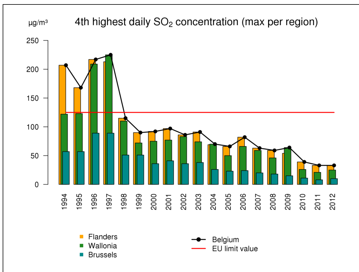
Figure 56 : évolution de la 4 ème concentration moyenne journalière de SO 2 maximale par Région et en Belgique sur base de la technique d'interpolation RIO.
