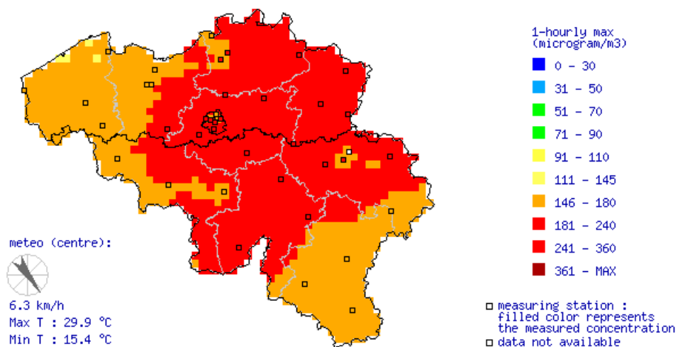
Figure 6: concentrations d'ozone horaires maximales le 25 juillet 2012.
