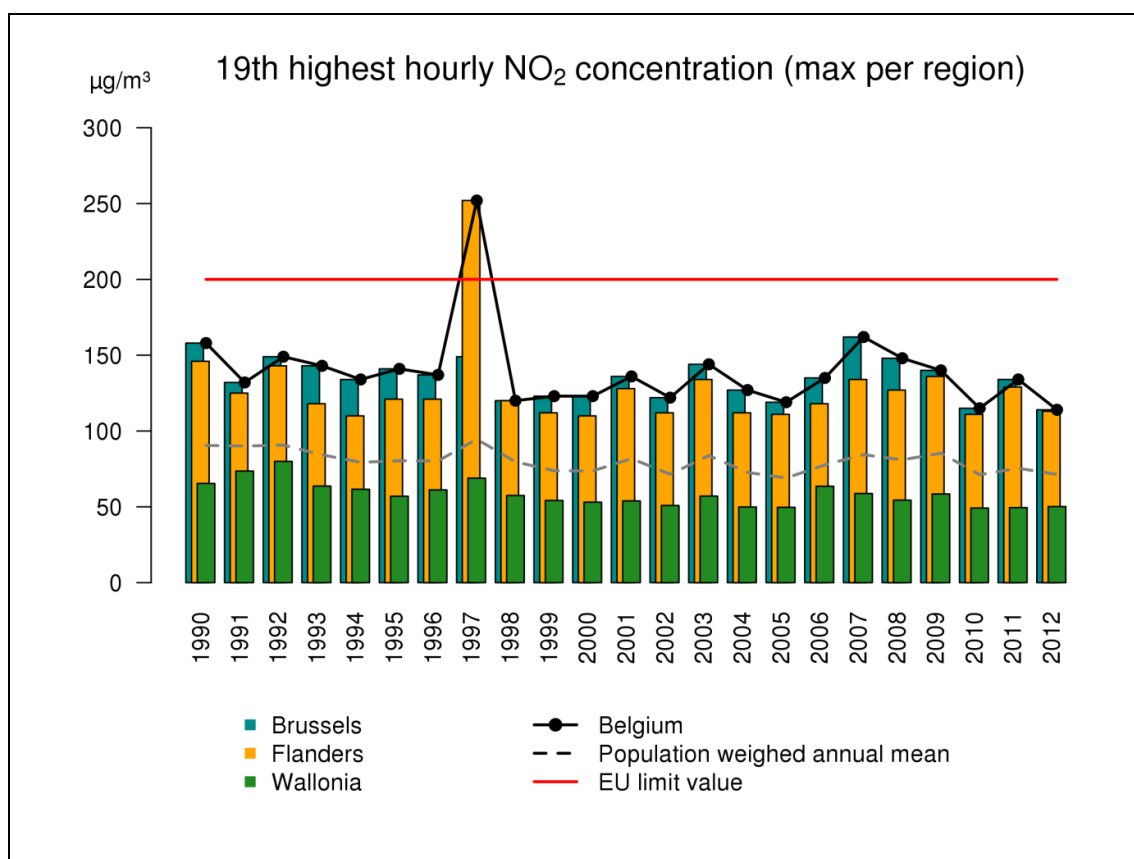
Figure 34 : évolution du maximum de la 19 ème valeur horaire la plus élevée de NO 2 dans les trois Régions et en Belgique, calculée sur base de la technique d'interpolation RIO.
