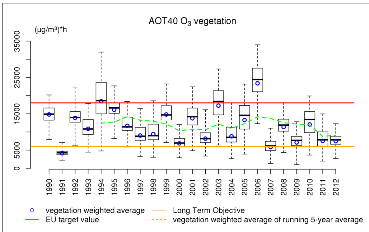
Figure 44: diagramme en boîtes de la surcharge pour la végétation (AOT40) en Belgique (1990-2012). Les moyennes pondérées en fonction de la végétation pour la Belgique sont représentées par les cercles bleus. La ligne pointillée verte indique la moyenne pondérée en fonction de la végétation de l'AOT40 sur 5 ans. Toutes les données ont été calculées sur base de la technique d'interpolation RIO.
