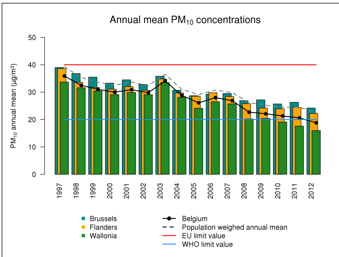
Figure 10: évolution de la concentration moyenne annuelle spatiale de PM 10 en Belgique et dans les trois Régions, et de la moyenne pondérée en fonction de la population pour la Belgique. Toutes les données ont été calculées sur base de la technique d'interpolation RIO.
