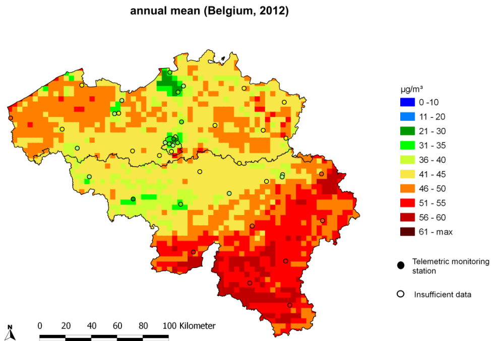
Figure 47: distribution spatiale de la concentration moyenne annuelle de O 3 en Belgique en 2012. « Insuffisant » signifie que les données ne respectent pas les critères établis dans l'annexe VII de la 2008/50/CE pour l'agrégation des données de mesure. Toutes les données ont été calculées sur base de la technique d'interpolation RIO.
